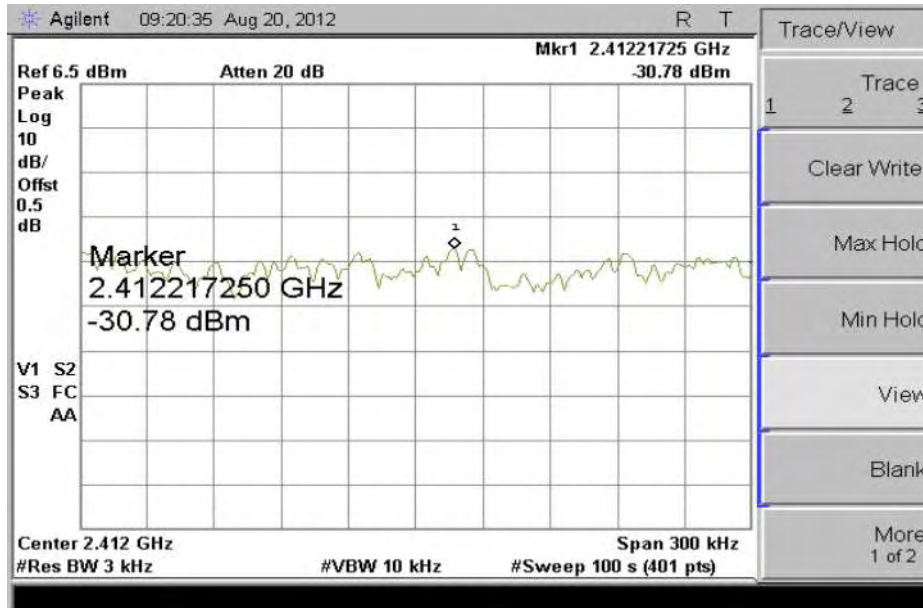
Plot - 802.11b-2412MHz
