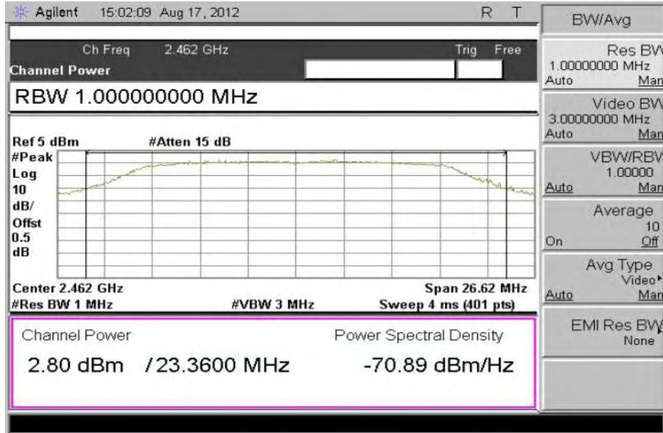
Plot - 802.11n-20Mhz-2462MHz
