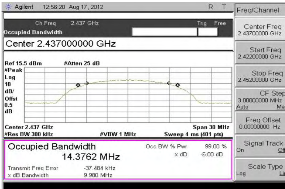
Plot - 802.11b-2437MHz
