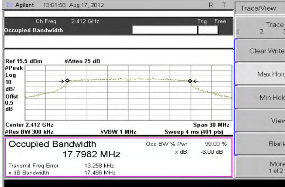
Plot - 802.11n-20MHz-2412MHz
