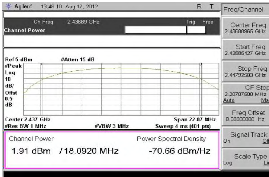
Plot - 802.11b-2437MHz
