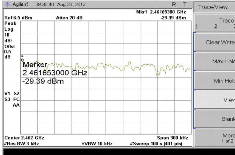
Plot - 802.11b-2462MHz
