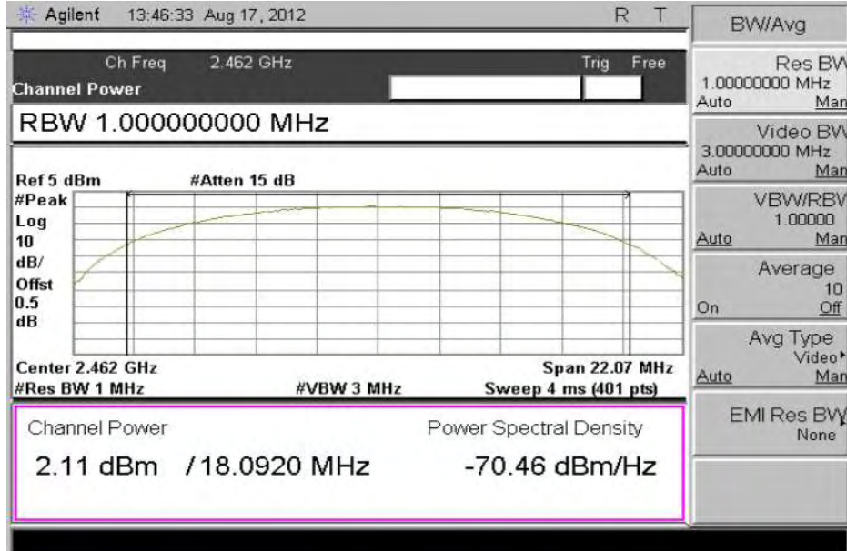
Plot - 802.11b-2462MHz
