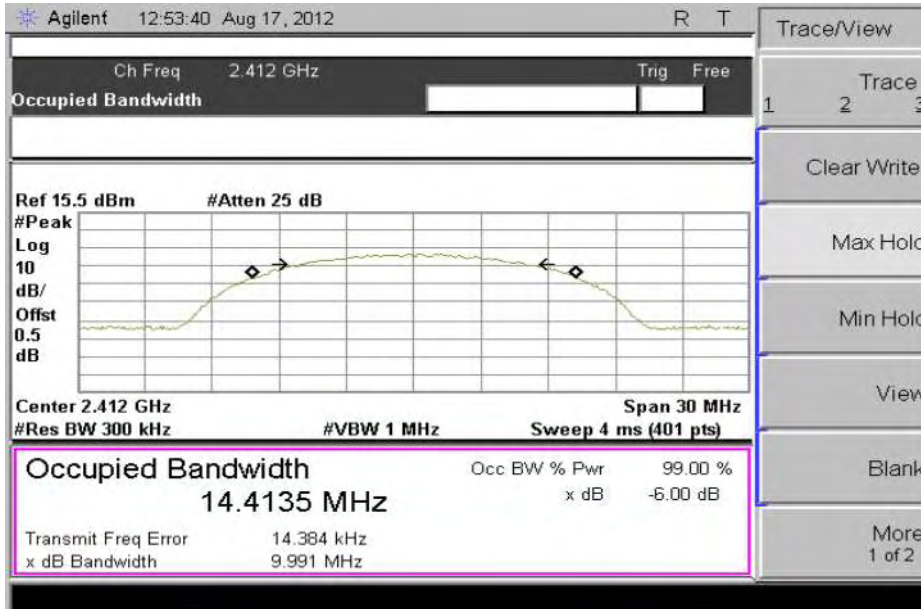
Plot - 802.11b-2412MHz
