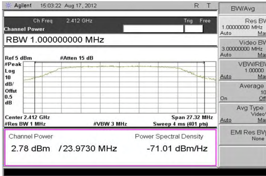
Plot - 802.11n-20MHz-2412MHz
