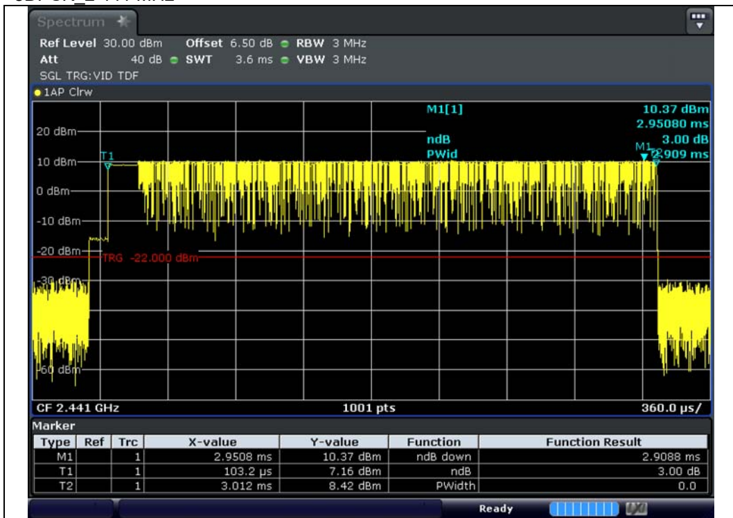
8DPSK 2 441 MHz
