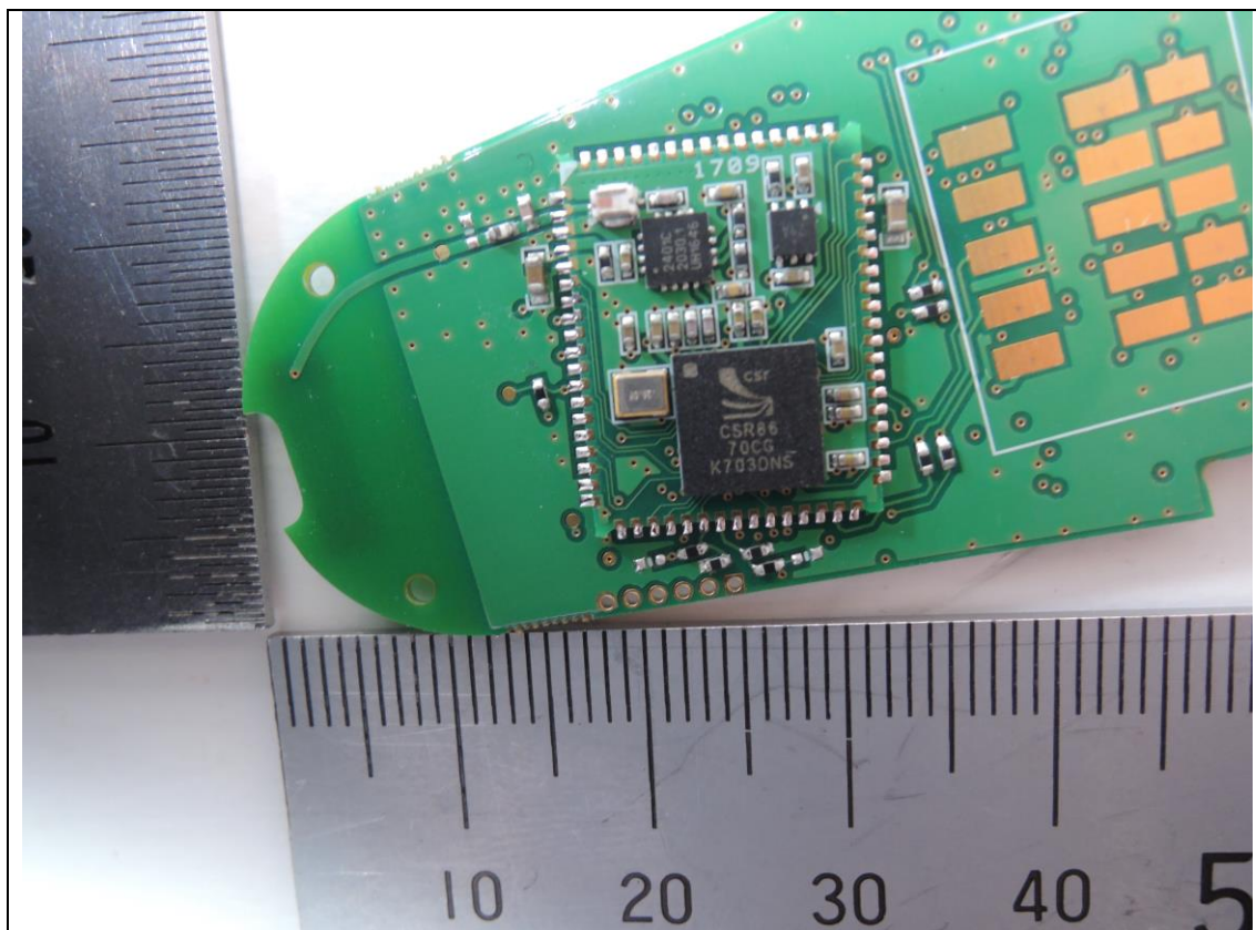
<Moudule>
