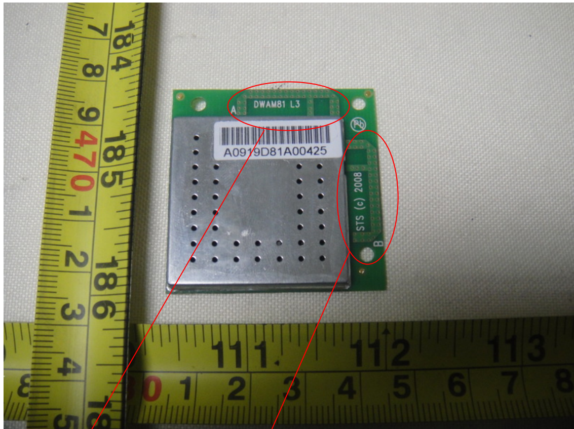
Antenna A
