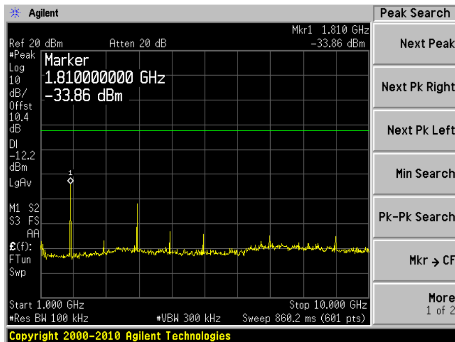
Plot: 1 – 10 GHz
