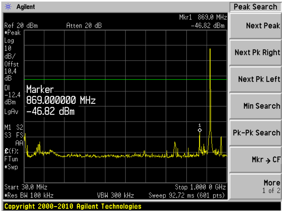
Plot: 30 MHz – 1 GHz
