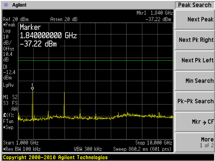
Plot: 1 – 10 GHz
