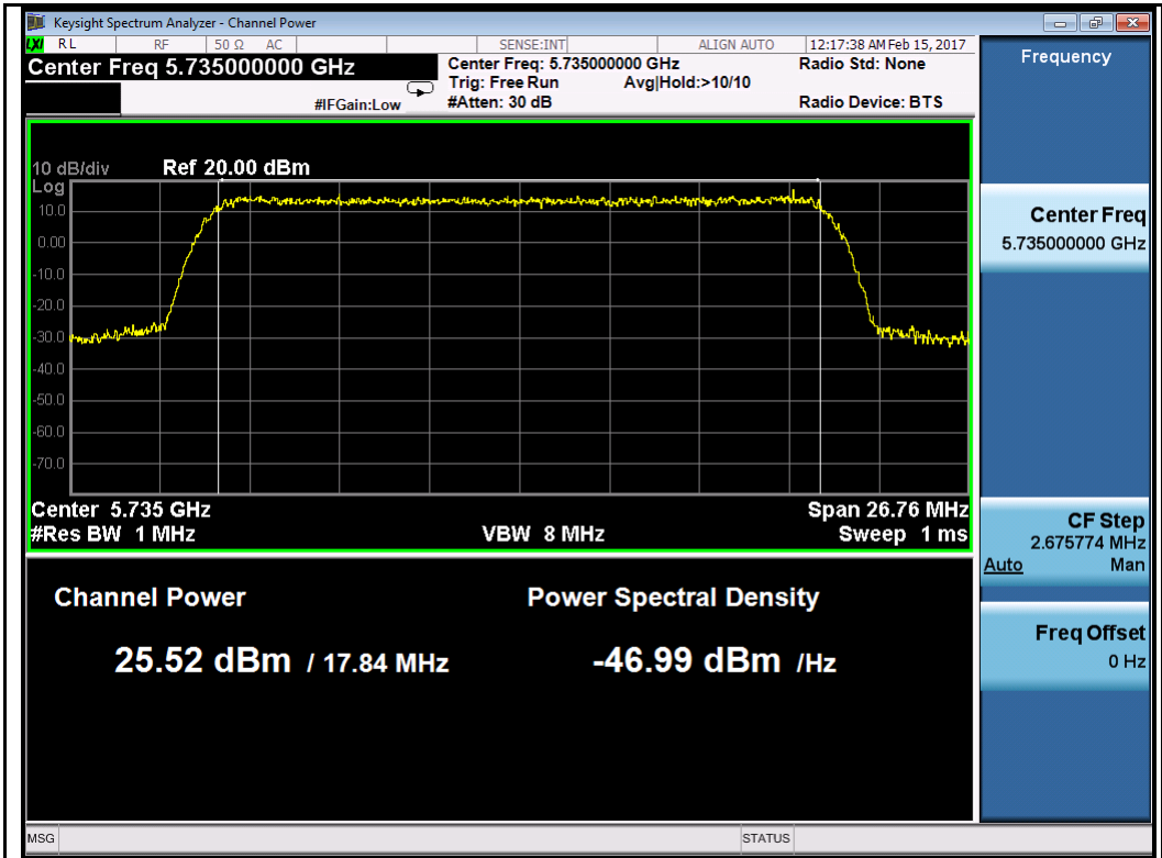
QPSK-5735MHz
