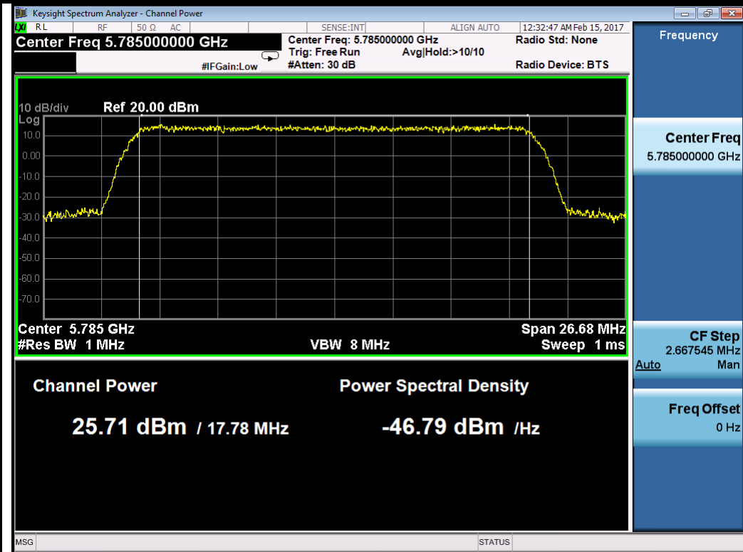
64QAM-5785MHz
