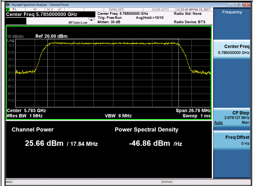
QPSK-5785MHz
