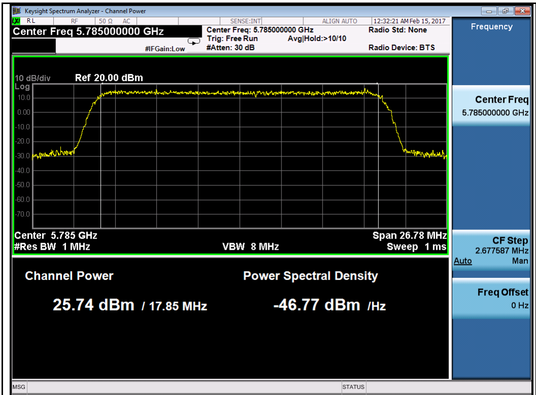
64QAM-5785MHz
