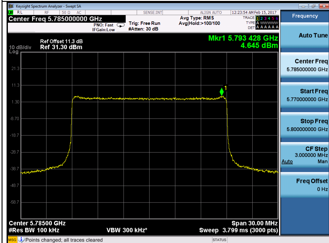
QPSK-5785MHz
