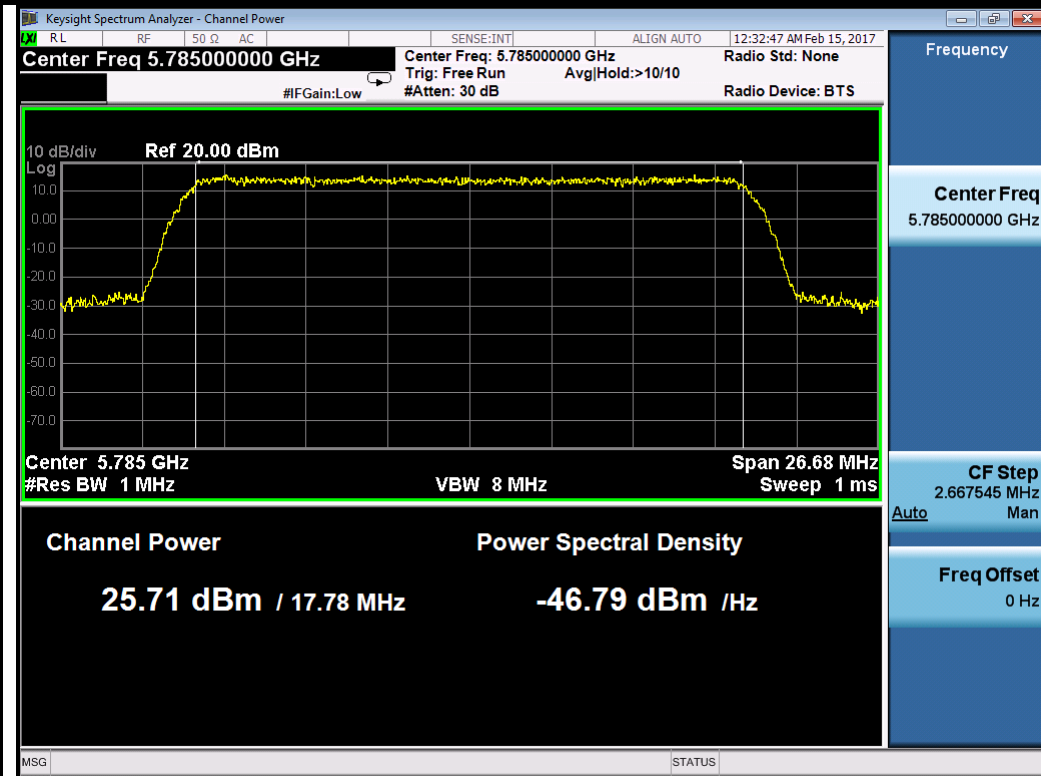
64QAM-5785MHz
