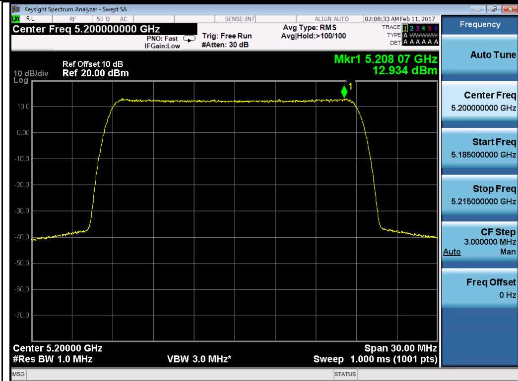
64QAM-5200MHz
