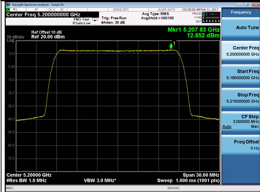
64QAM-5200MHz
