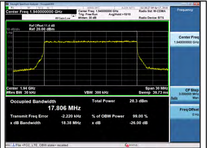
OBW- Band2 -20M BW-Low
