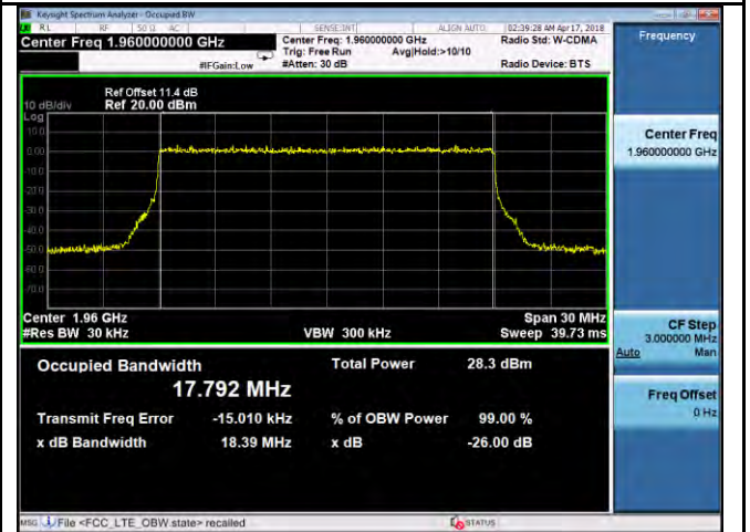
OBW- Band2-20M BW-Mid
