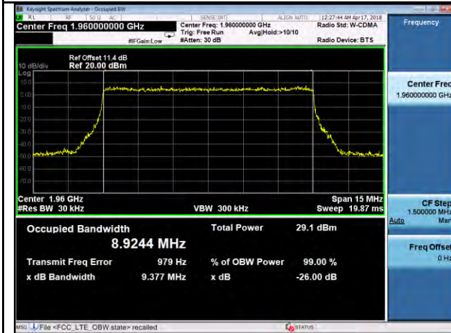
OBW- Band2 -10M BW-Mid
