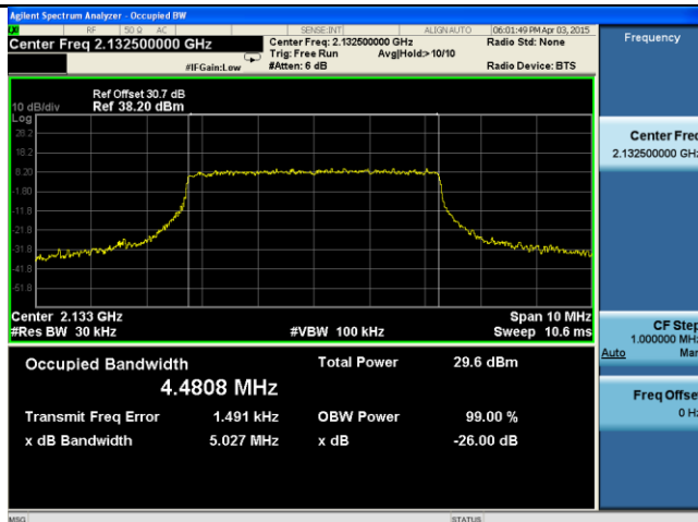
OBW-Band4-5M BW-Mid
