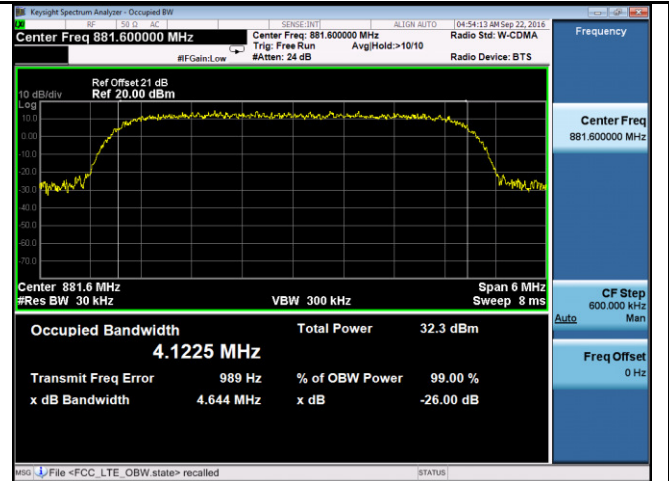
OBW- Band5-Mid
