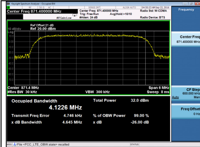
OBW- Band5-Low
