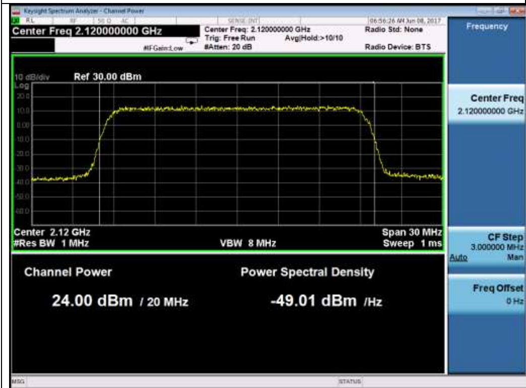
20M QPSK Low
