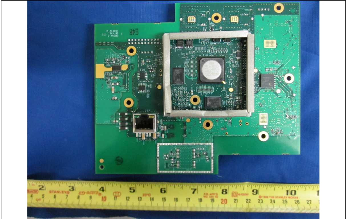
EUT – bottom
