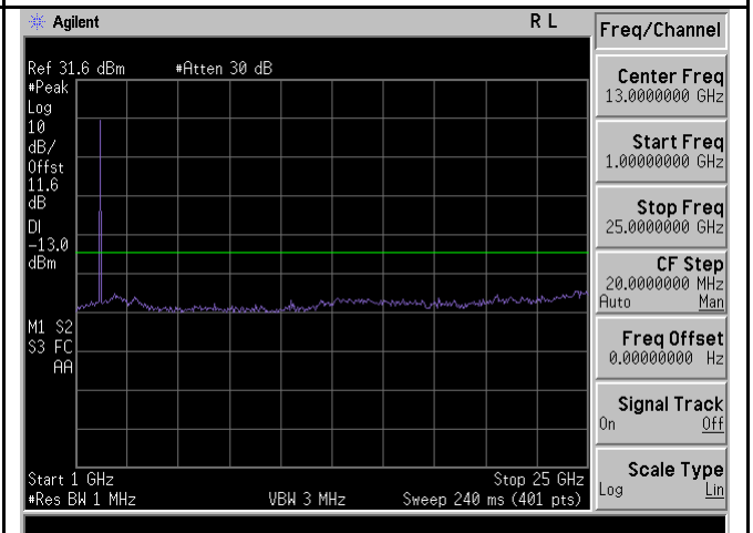
TX CSE-Band4-QPSK-5M BW-Mid CH-above 1G
