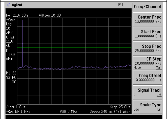
TX CSE-Band4-QPSK-10M BW-Mid CH-above 1G
