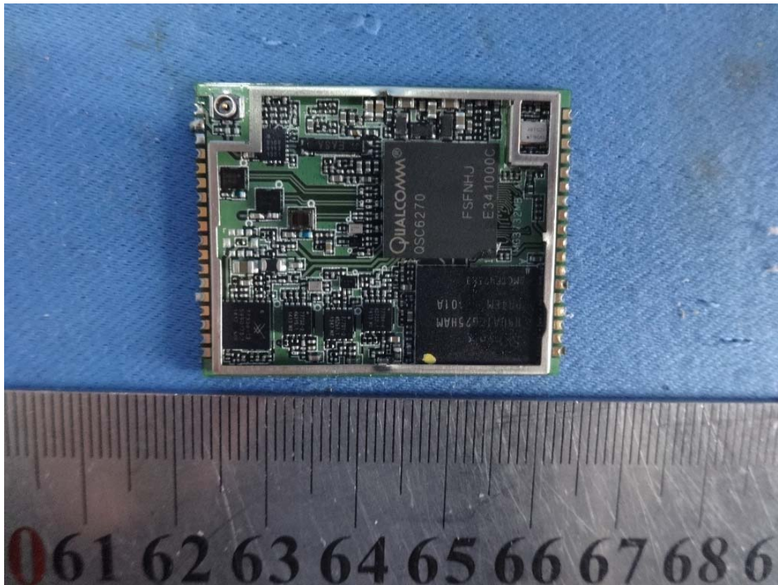
3G Module:
