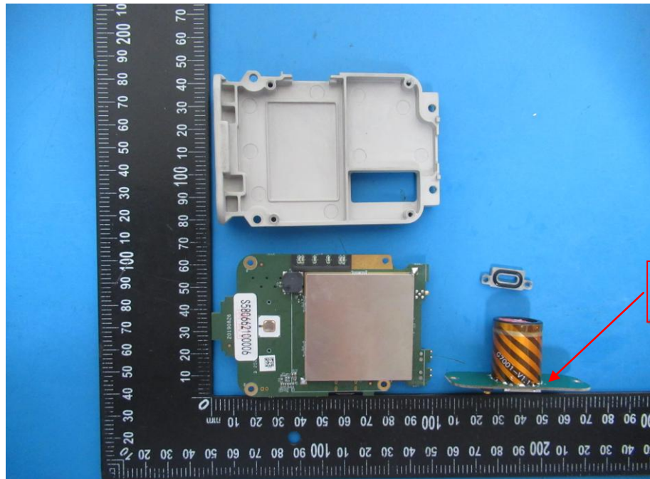
Antenna
