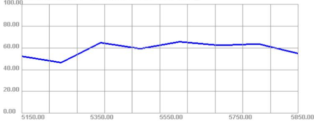
5150.00MHz - 5850.00MHz Efficiency
