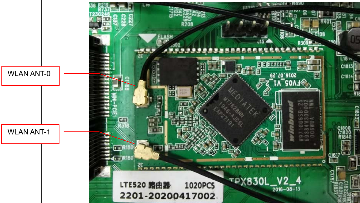
EUT Photo (6)
