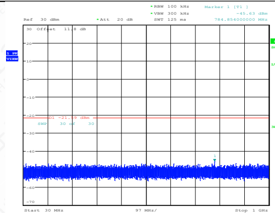
BLE_2M-Ant1-2440-30~1000-PASS
