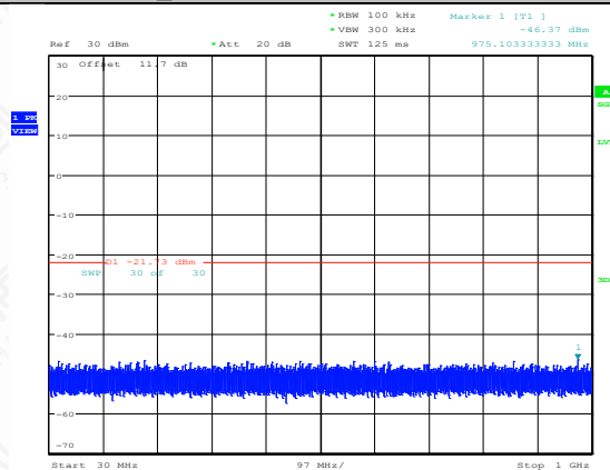
BLE_2M-Ant1-2480-30~1000-PASS
