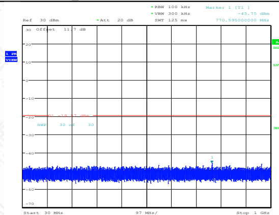
BLE_2M-Ant1-2402-30~1000-PASS
