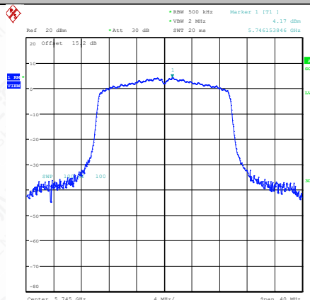
11AX20MIMO-Ant1-5745-PASS
