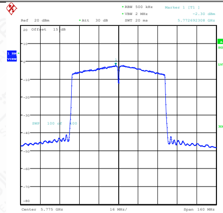
11AC80SISO-Ant2-5775-PASS
