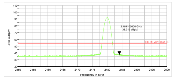
BLE Channel 39 Average
