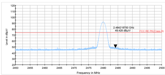
BLE Channel 39 Peak
