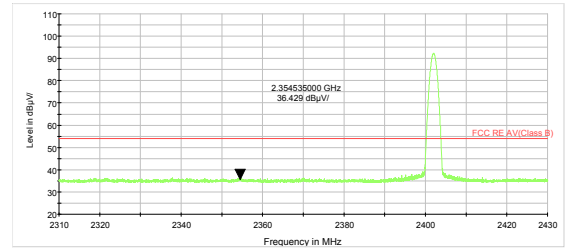
BLE Channel 0 Average
