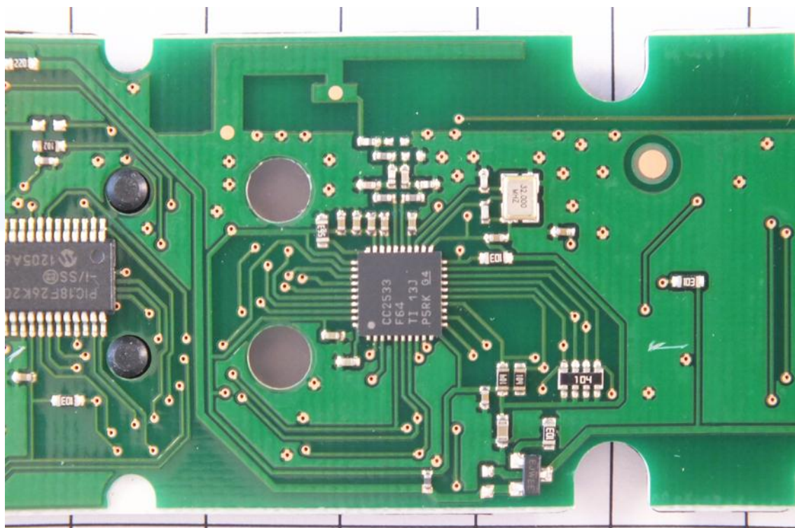
PCB-Antenna
