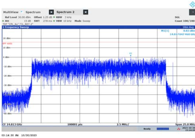
f_{LOW} (19.8 MHz, QPSK)
