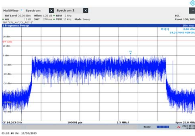
f_{MID} (19.8 MHz, QPSK)
