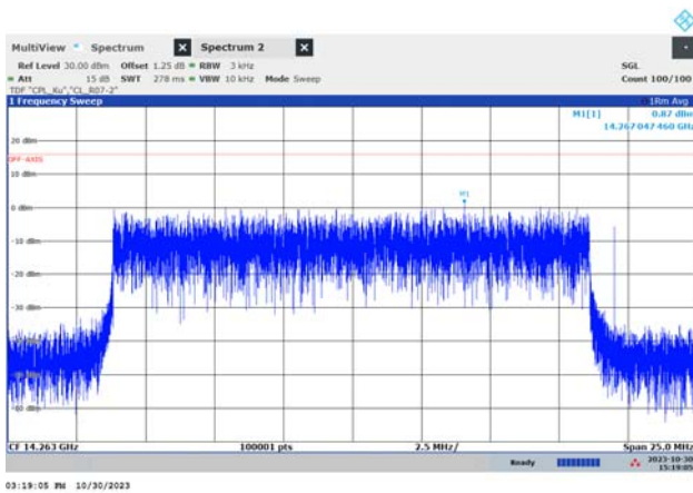
f_{MID} (19.8 MHz, 8PSK)
