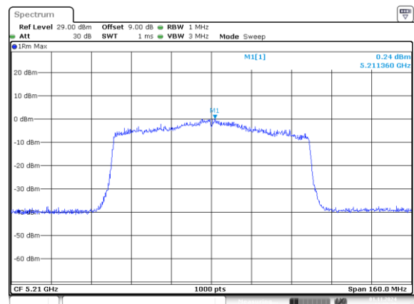
802.11ax80_5210MHz_RU_996/67_Chain 1
