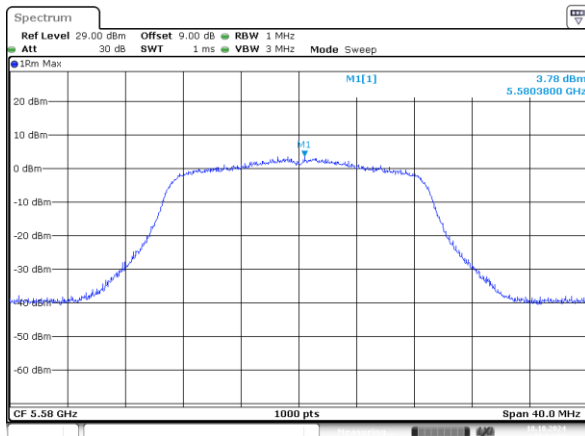
802.11n20_5580MHz_Chain 0
