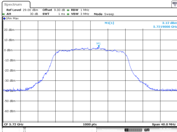
802.11a_5720MHz_Chain 0
