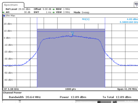
802.11n20_5580MHz_Chain 0
