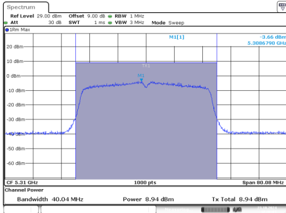
802.11n40_5310MHz_Chain 0
