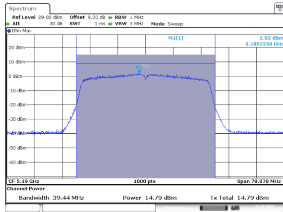
802.11n40_5190MHz_Chain 0
