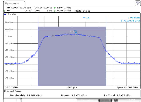
802.11n20_5700MHz_Chain 1
