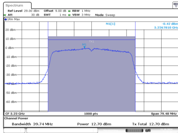
802.11n40_5230MHz_Chain 0
