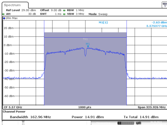
802.11ac160_5570MHz_Chain 0
