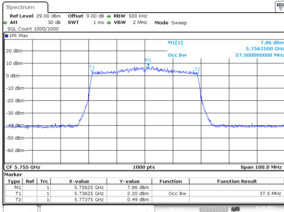
802.11ax40_5755MHz_RU_484/65_Chain 0 37.500MHz
