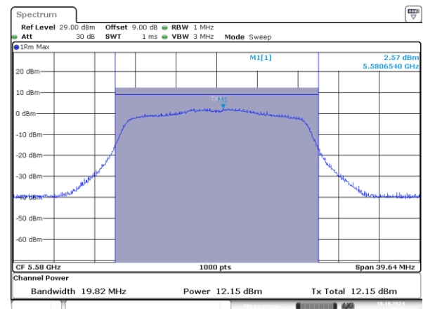
802.11n20_5580MHz_Chain 1
