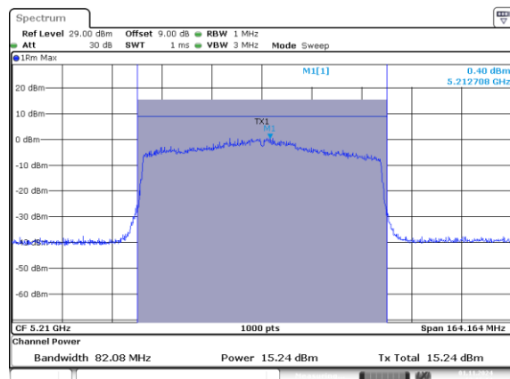
802.11ax80_5210MHz_RU_996/67_Chain 0
