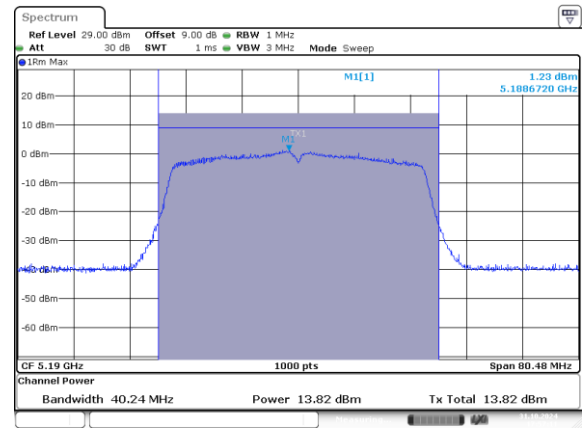
802.11n40_5190MHz_Chain 1
