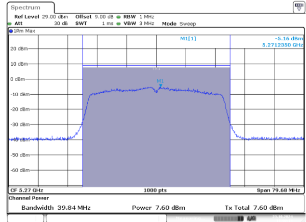
802.11n40_5270MHz_Chain 1
