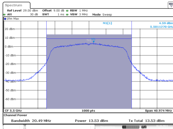
802.11n20_5500MHz_Chain 0
