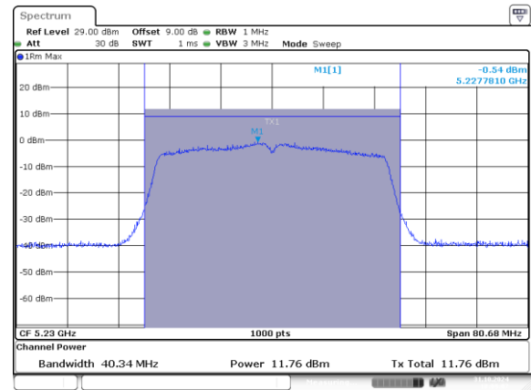
802.11n40_5230MHz_Chain 1
