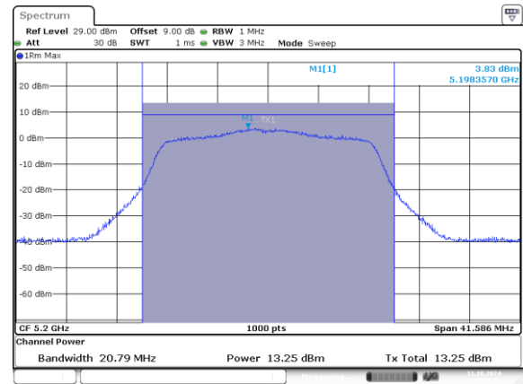
802.11n20_5200MHz_Chain 1
