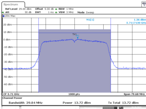
802.11n40_5710MHz_Chain 0
