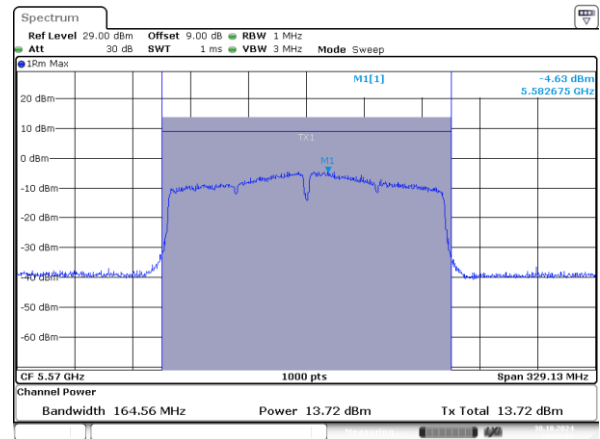
802.11ac160_5570MHz_Chain 1
