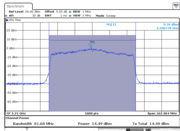
802.11ax80_5210MHz_RU_996/67_Chain 1
