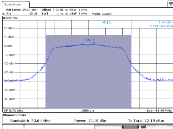
802.11n20_5720MHz_Chain 0
