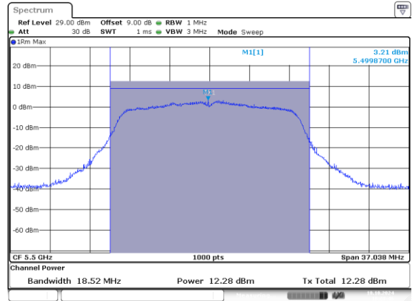
802.11a_5500MHz_Chain 1
