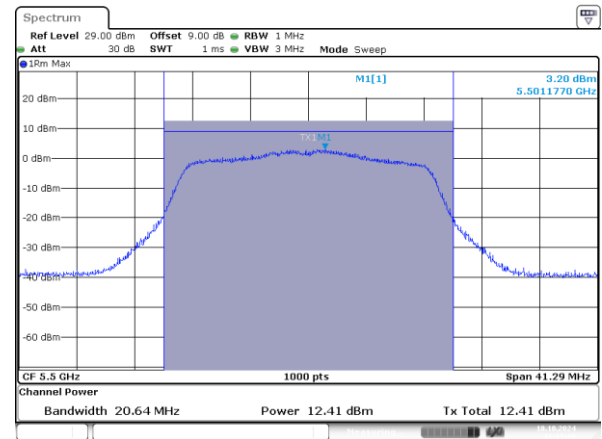
802.11n20_5500MHz_Chain 1
