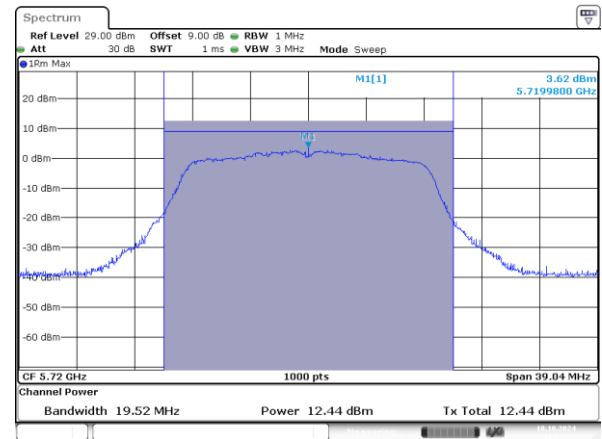
802.11a_5720MHz_Chain 1
