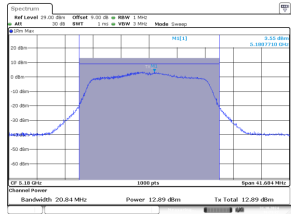
802.11n20_5180MHz_Chain 1
