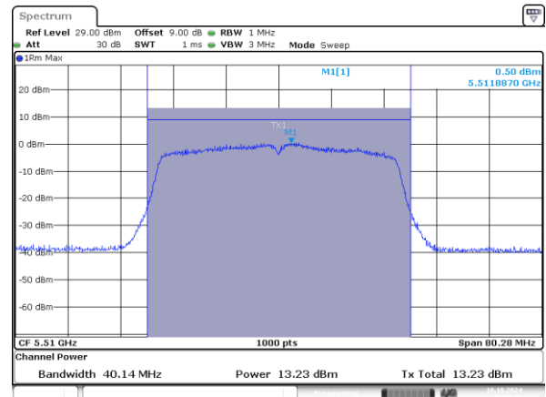
802.11n40_5510MHz_Chain 1
