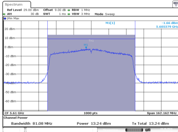
802.11ac80_5610MHz_Chain 0
