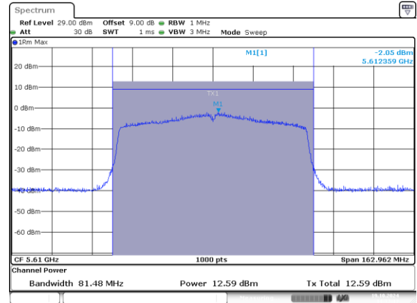
802.11ac80_5610MHz_Chain 1
