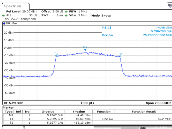
802.11ac80_5290MHz_Chain 0 75.200MHz
