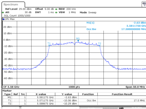
802.11n20_5580MHz_Chain 0 17.500MHz
