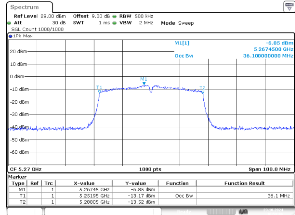
802.11n40_5270MHz_Chain 1 36.100MHz
