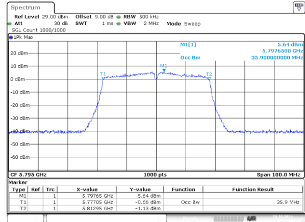
802.11n40_5795MHz_Chain 1 35.900MHz
