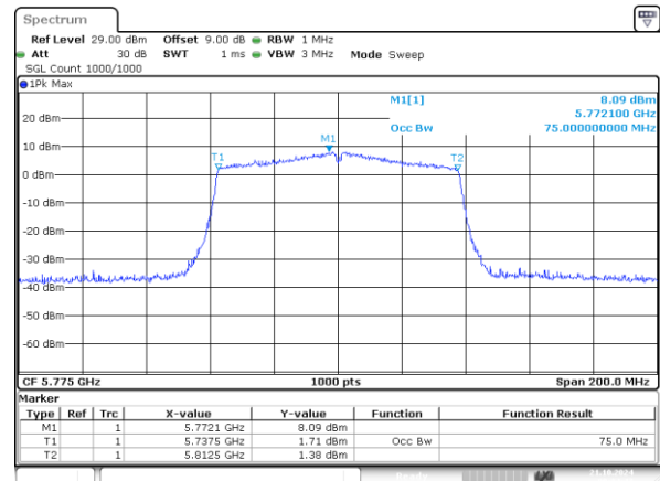
802.11ac80_5775MHz_Chain 1 75MHz
