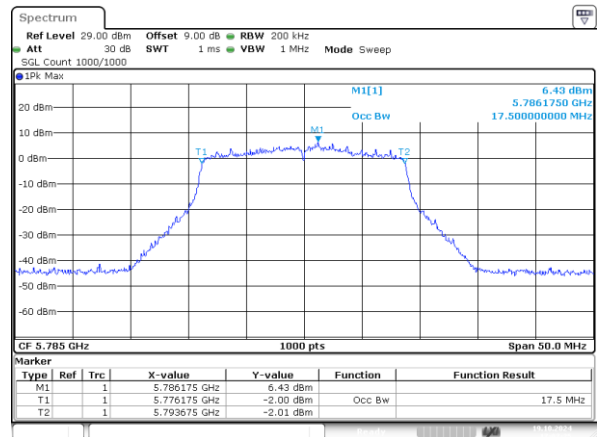
802.11n20_5785MHz_Chain 1 17.500MHz
