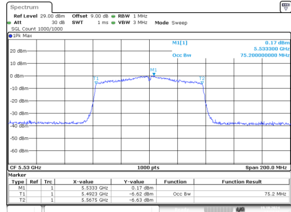
802.11ac80_5530MHz_Chain 1 75.200MHz
