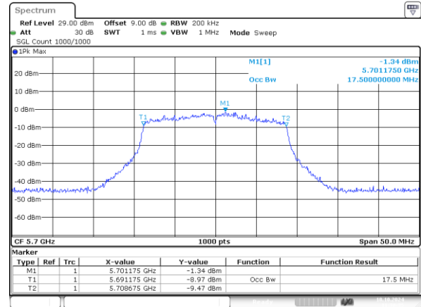
802.11n20_5700MHz_Chain 1 17.500MHz
