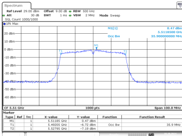
802.11n40_5510MHz_Chain 0 35.900MHz
