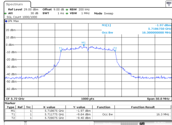
802.11a_5720MHz_Chain 1 16.300MHz
