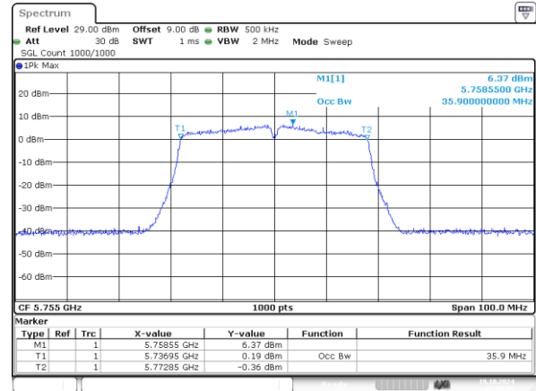
802.11n40_5755MHz_Chain 1 35.900MHz
