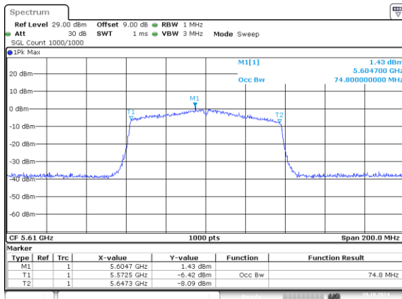
802.11ac80_5610MHz_Chain 0 74.800MHz
