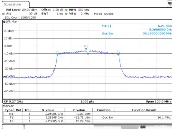
802.11n40_5270MHz_Chain 0 36.100MHz
