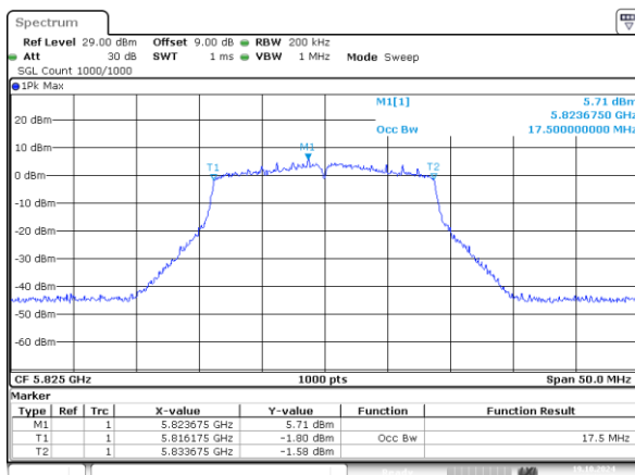
802.11n20_5825MHz_Chain 0 17.500MHz
