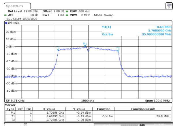
802.11n40_5710MHz_Chain 1 35.900MHz
