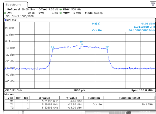
802.11n40_5310MHz_Chain 1 36.100MHz
