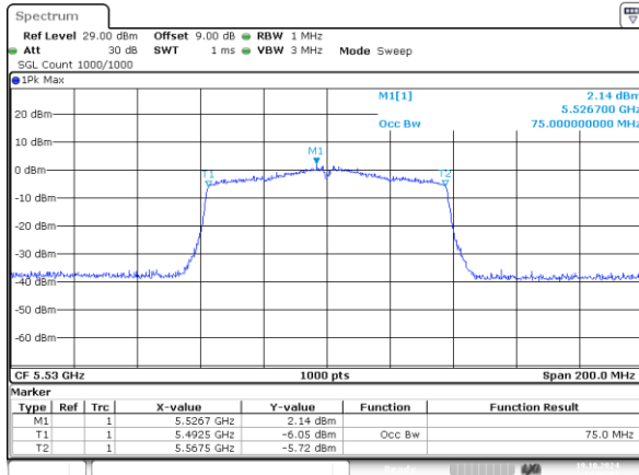
802.11ac80_5530MHz_Chain 0 75MHz
