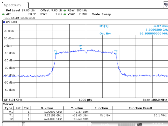
802.11n40_5310MHz_Chain 0 36.100MHz
