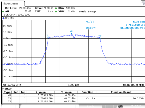
802.11n40_5755MHz_Chain 0 36MHz
