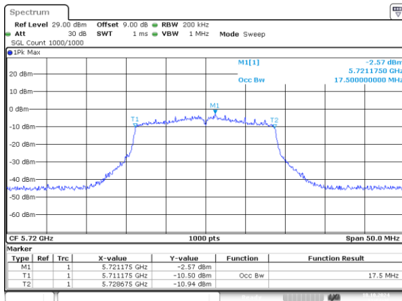
802.11n20_5720MHz_Chain 0 17.500MHz
