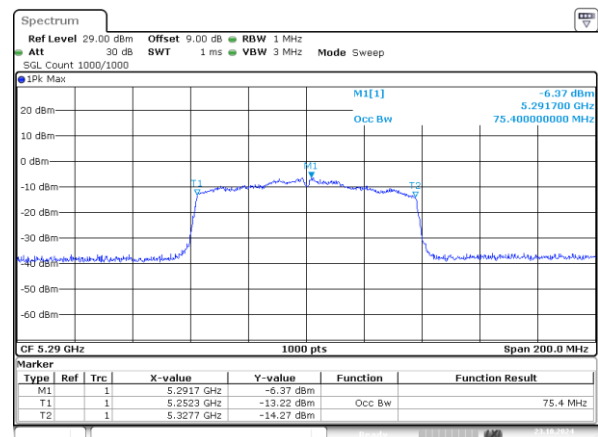
802.11ac80_5290MHz_Chain 1 75.400MHz
