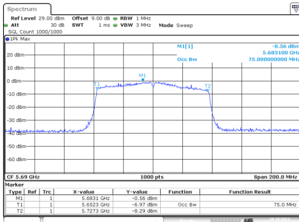
802.11ac80_5690MHz_Chain 0 75MHz
