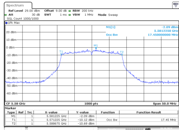
802.11n20_5580MHz_Chain 1 17.450MHz
