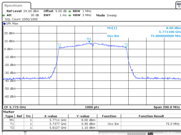
802.11ac80_5775MHz_Chain 0 75MHz
