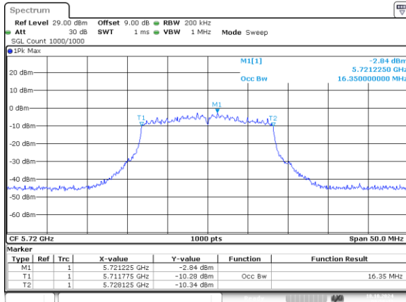
802.11a_5720MHz_Chain 0 16.350MHz
