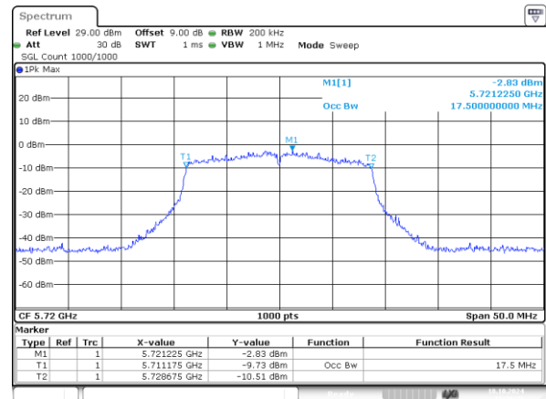
802.11n20_5720MHz_Chain 1 17.500MHz
