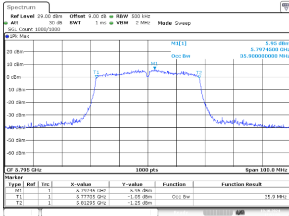
802.11n40_5795MHz_Chain 0 35.900MHz
