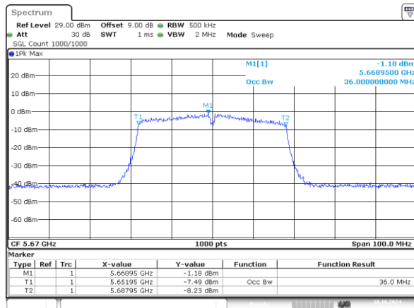
802.11n40_5670MHz_Chain 0 36MHz
