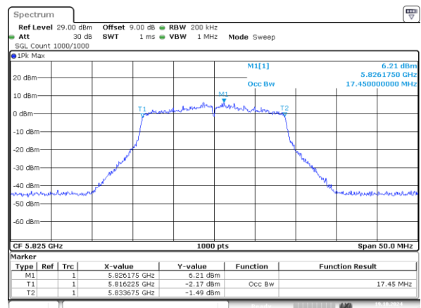
802.11n20_5825MHz_Chain 1 17.450MHz
