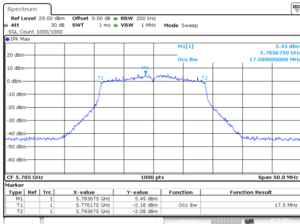
802.11n20_5785MHz_Chain 0 17.500MHz
