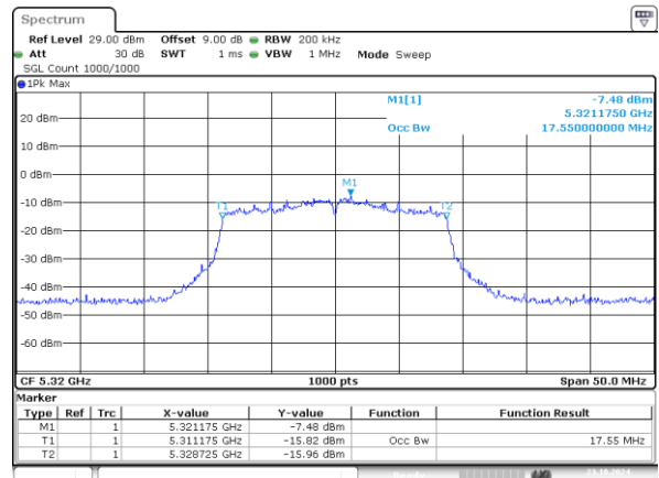
802.11n20_5320MHz_Chain 1 17.550MHz
