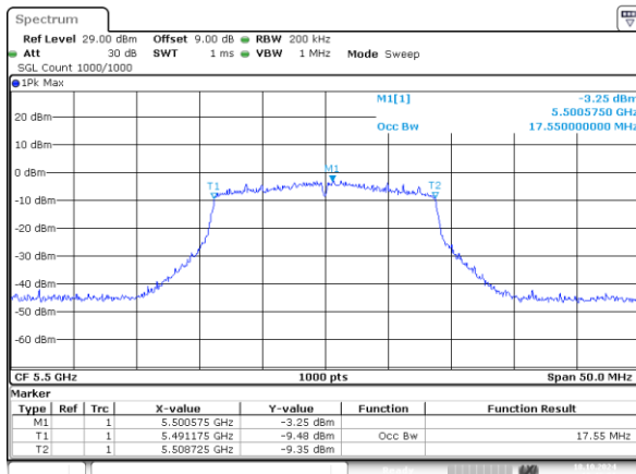
802.11n20_5500MHz_Chain 0 17.550MHz
