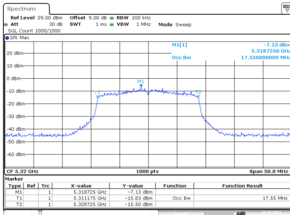
802.11n20_5320MHz_Chain 0 17.550MHz
