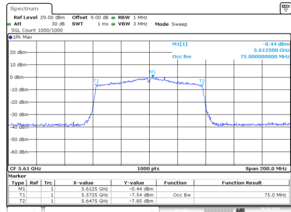
802.11ac80_5610MHz_Chain 1 75MHz
