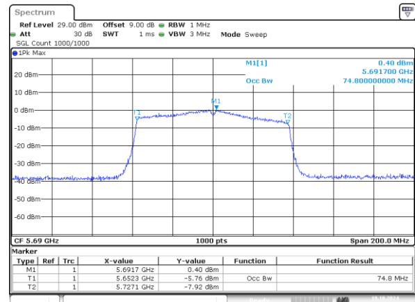
802.11ac80_5690MHz_Chain 1 74.800MHz
