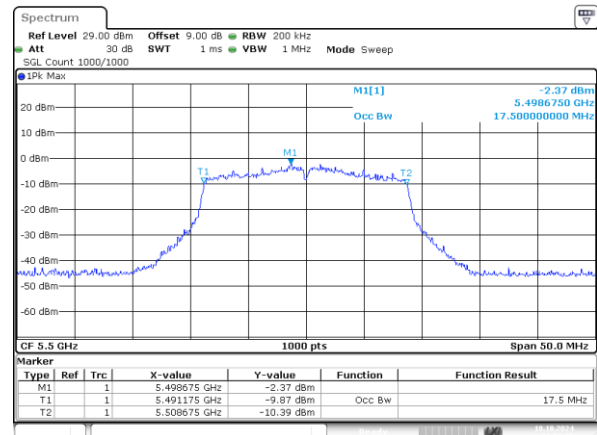
802.11n20_5500MHz_Chain 1 17.500MHz
