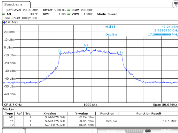
802.11n20_5700MHz_Chain 0 17.500MHz
