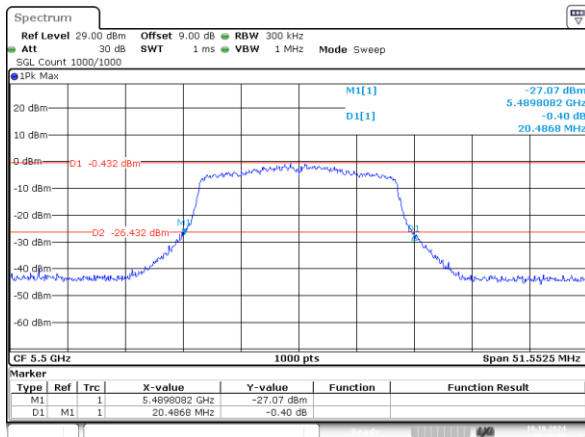
802.11n20_5500MHz_Chain 0 20.487MHz
