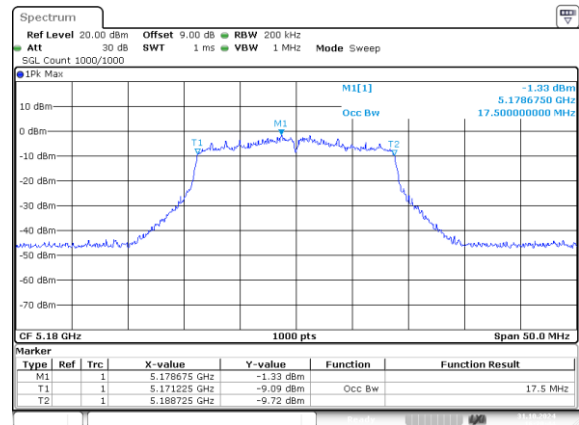
802.11n20_5180MHz_Chain 1 17.500MHz
