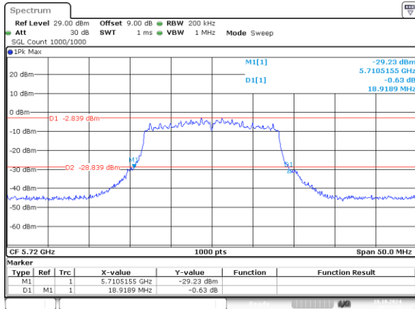
802.11a_5720MHz_Chain 0 18.919MHz
