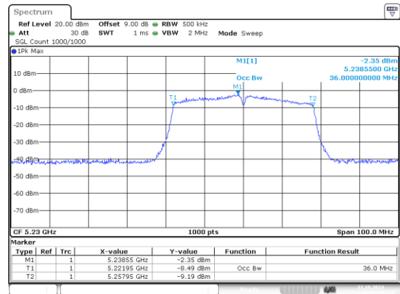
802.11n40_5230MHz_Chain 1 36MHz
