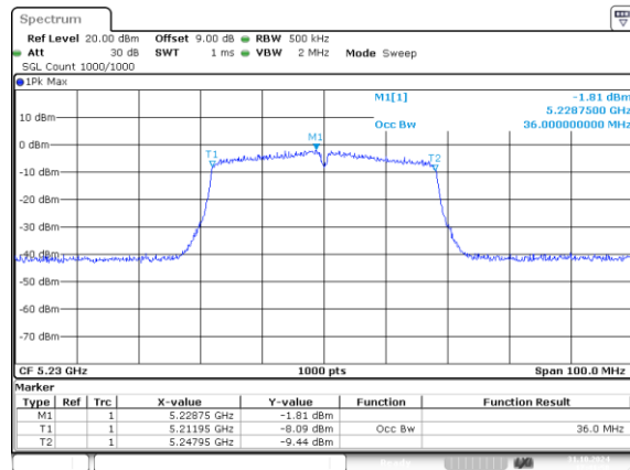
802.11n40_5230MHz_Chain 0 36MHz
