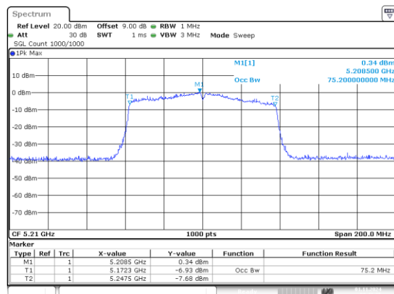
802.11ac80_5210MHz_Chain 0 75.200MHz
