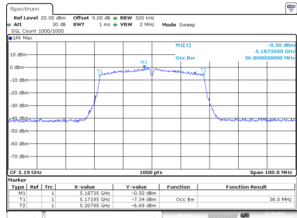
802.11n40_5190MHz_Chain 1 36MHz
