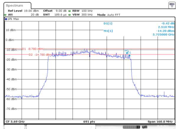
802.11ac80_5690MHz_Chain 1 2.510MHz
