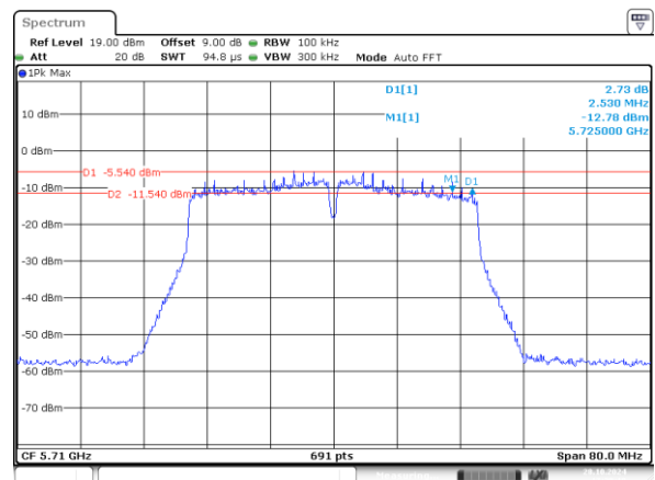
802.11n40_5710MHz_Chain 1 2.530MHz
