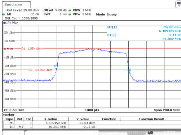
802.11ac80_5530MHz_Chain 0 81.882MHz
