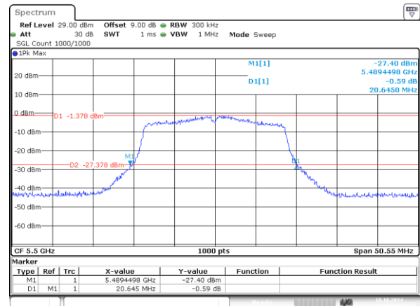
802.11n20_5500MHz_Chain 1 20.645MHz
