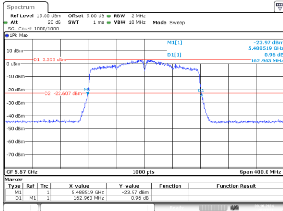
802.11ac160_5570MHz_Chain 0 162.963MHz
