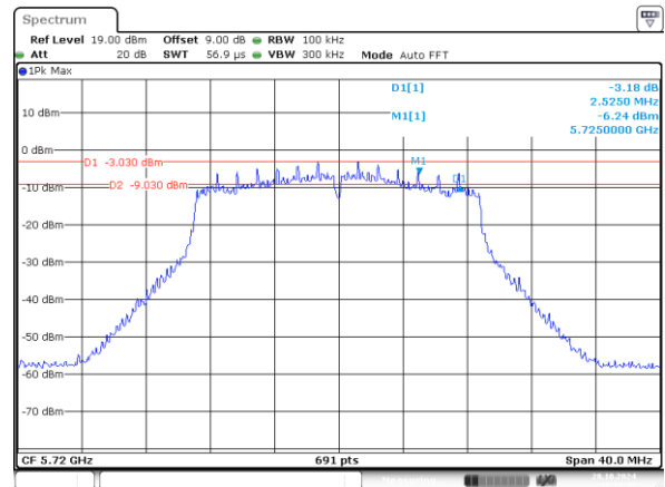
802.11n20_5720MHz_Chain 1 2.525MHz
