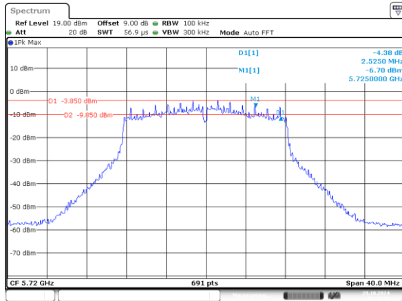
802.11a_5720MHz_Chain 0 2.525MHz
