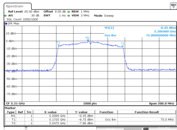
802.11ac80_5210MHz_Chain 1 75MHz
