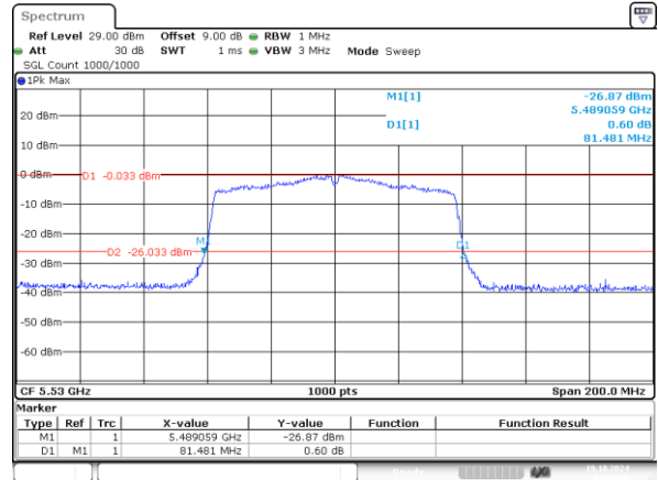
802.11ac80_5530MHz_Chain 1 81.481MHz
