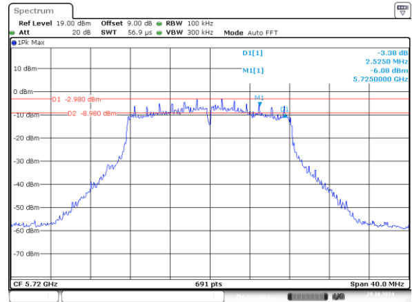
802.11a_5720MHz_Chain 1 2.525MHz
