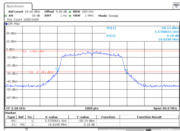
802.11n20_5580MHz_Chain 1 19.820MHz
