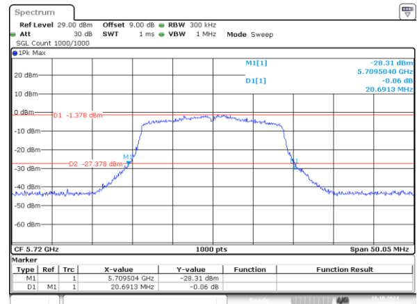
802.11n20_5720MHz_Chain 1 20.691MHz
