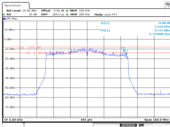
802.11ac80_5690MHz_Chain 0 2.510MHz
