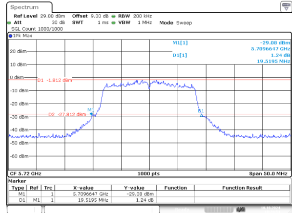
802.11a_5720MHz_Chain 1 19.520MHz
