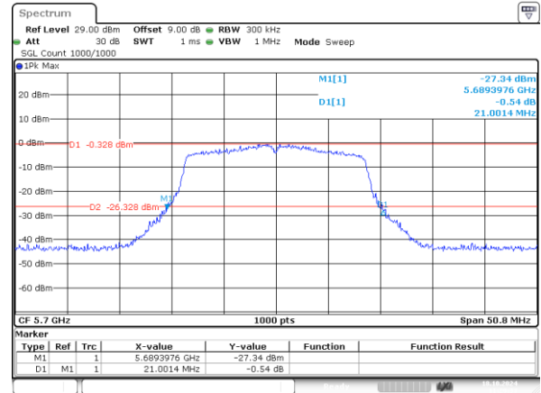
802.11n20_5700MHz_Chain 1 21.001MHz
