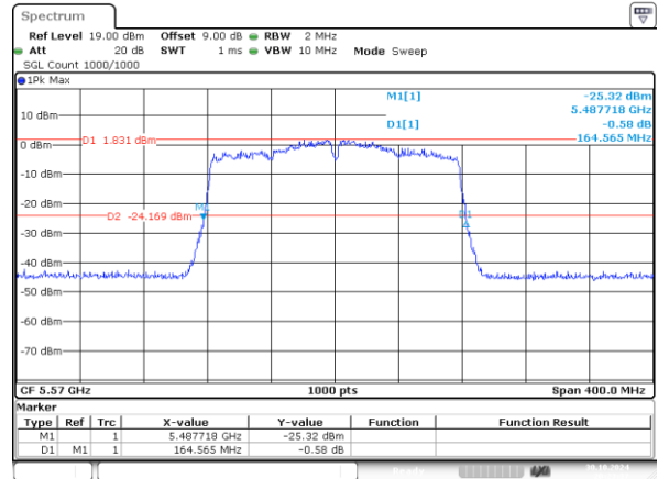
802.11ac160_5570MHz_Chain 1 164.565MHz
