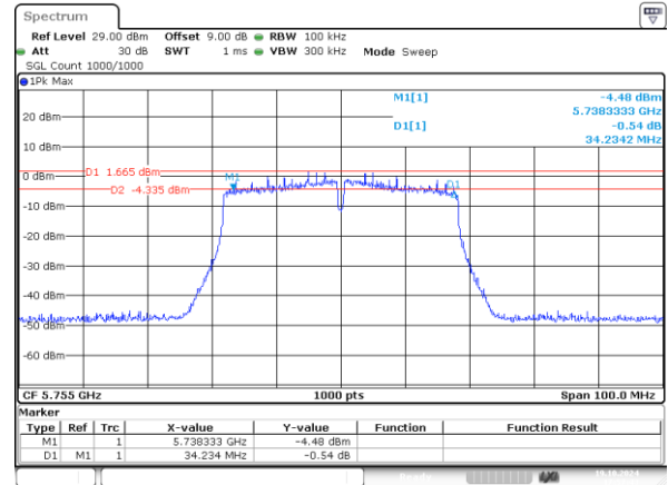
802.11n40_5755MHz_Chain 1 34.234MHz
