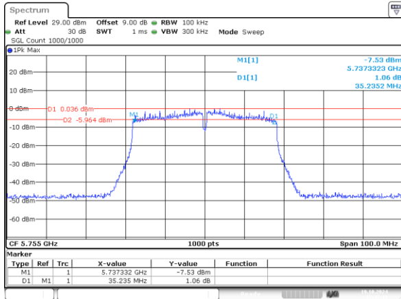
802.11n40_5755MHz_Chain 0 35.235MHz
