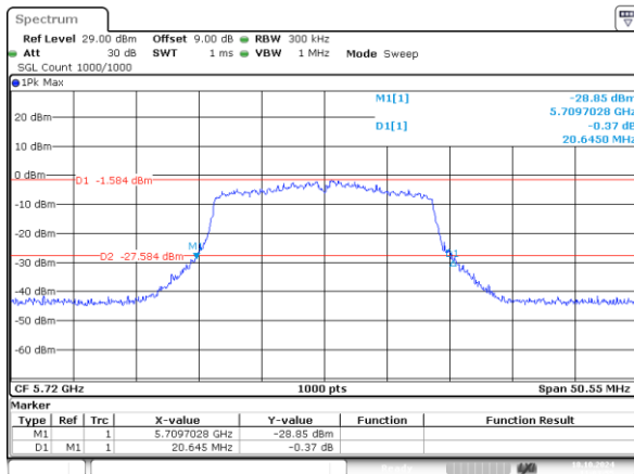
802.11n20_5720MHz_Chain 0 20.645MHz
