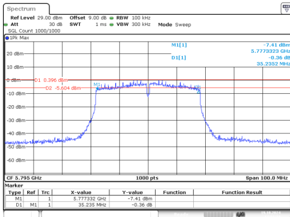
802.11n40_5795MHz_Chain 0 35.235MHz
