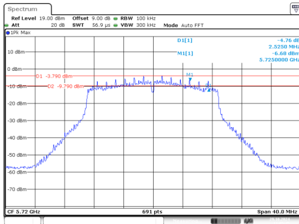
802.11n20_5720MHz_Chain 0 2.525MHz
