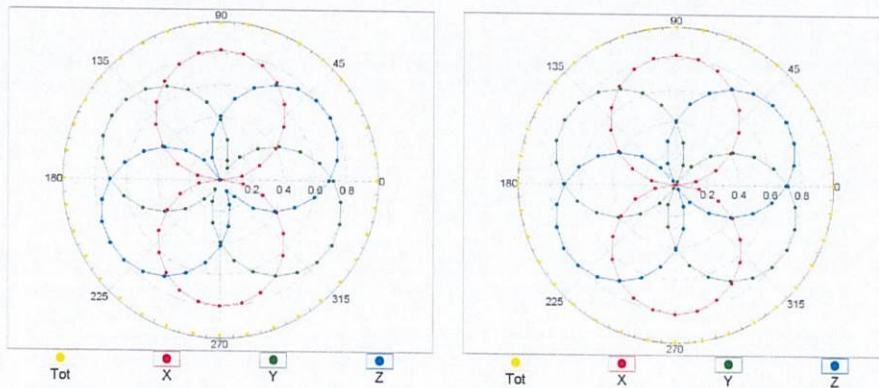
f=1800 MHz,R22
