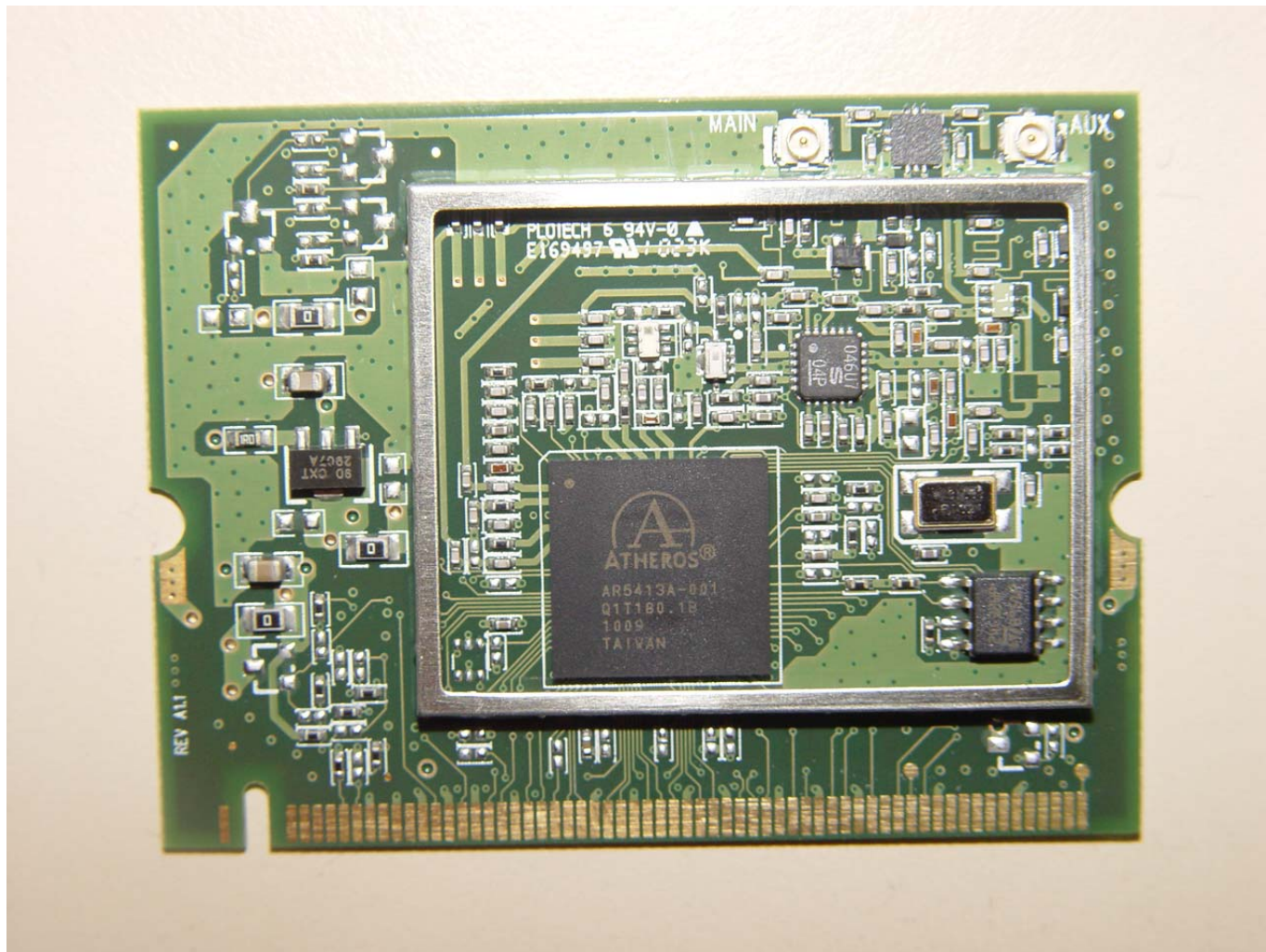
WiFi Module WLM54AG, top
