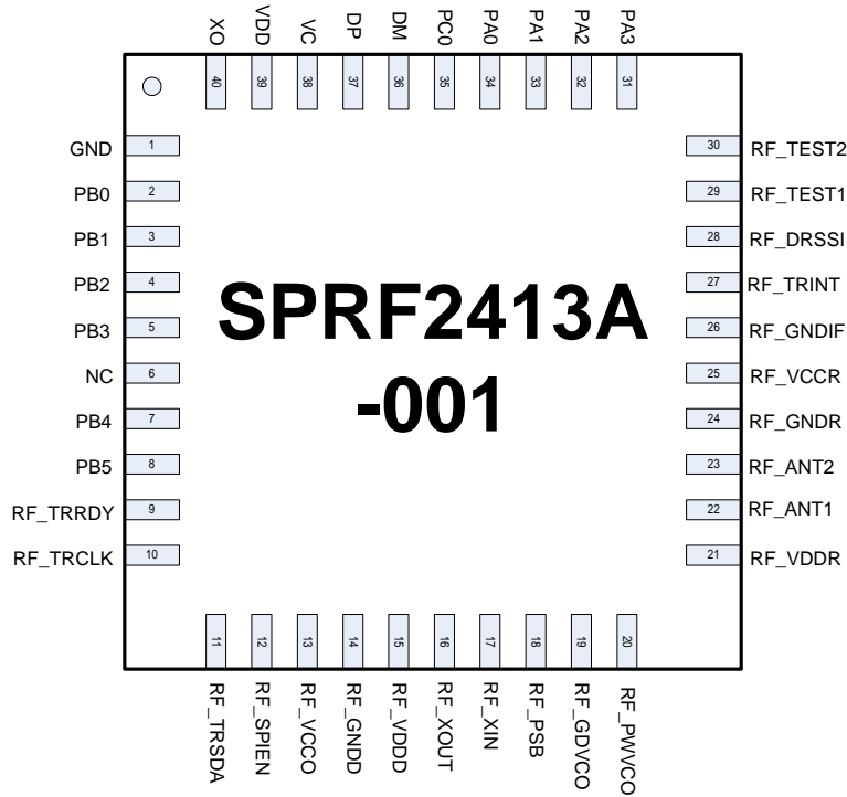
SPRF2413A-001 QFN40
