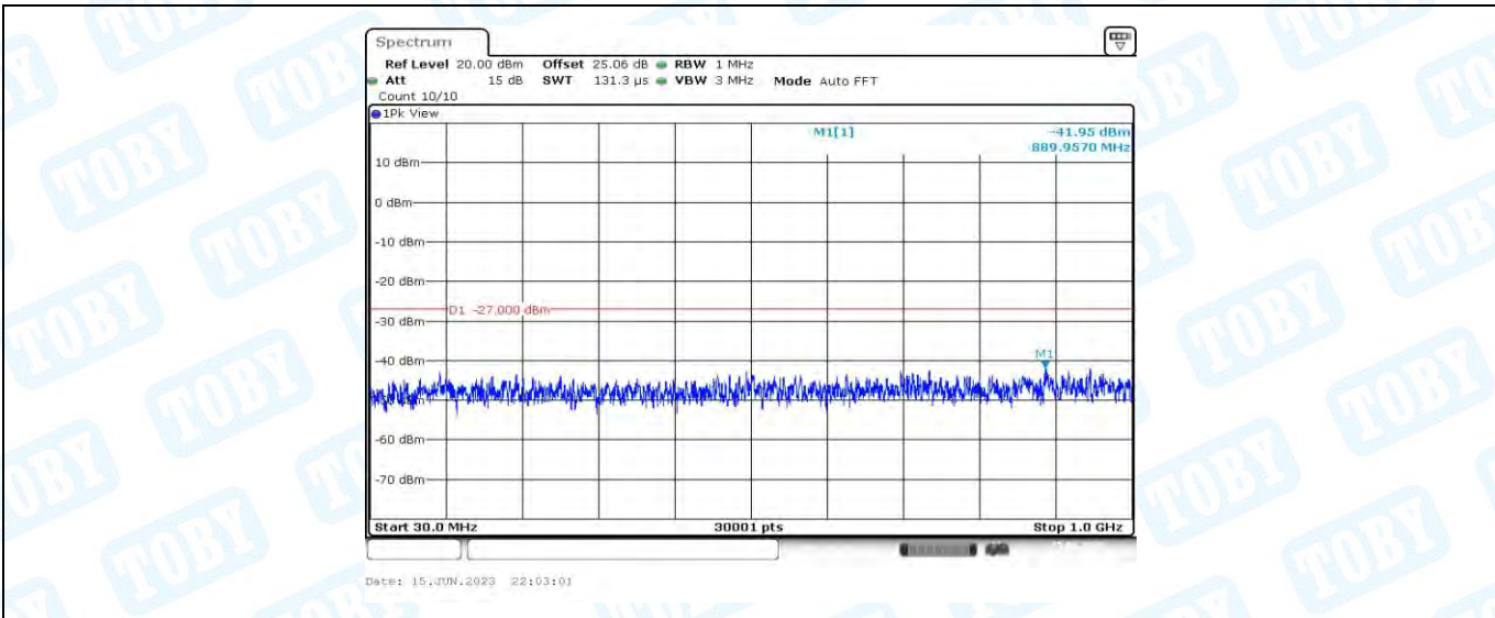
11AC20MIMO_Ant1_5500_30~1000
