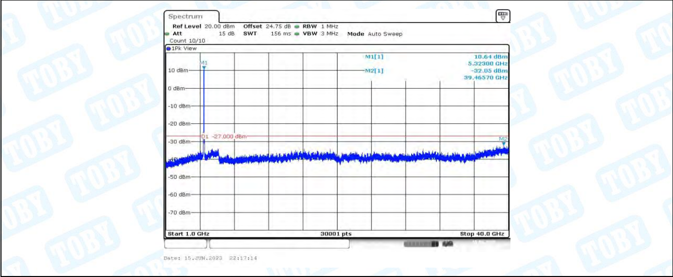
11AC40MIMO_Ant2_5310_1000~40000
