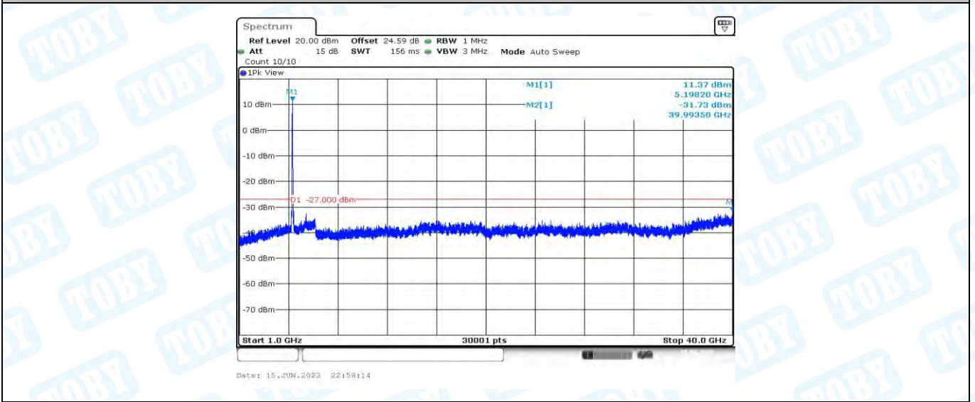
11AX40MIMO_Ant2_5190_1000~40000
