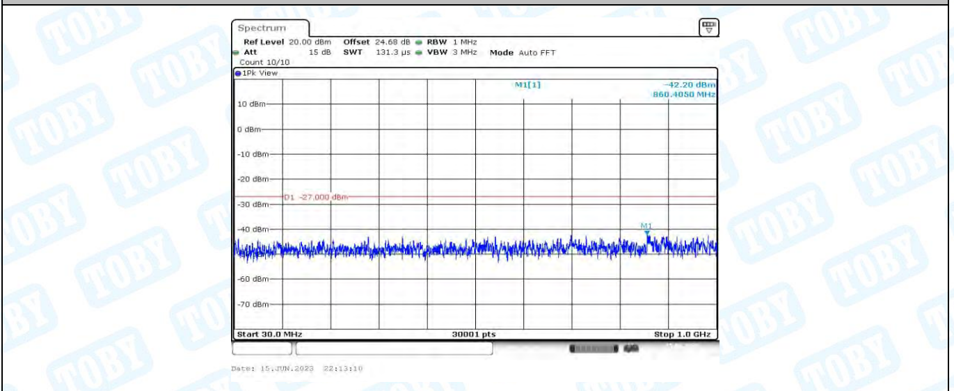
11AC40MIMO_Ant1_5230_30~1000
