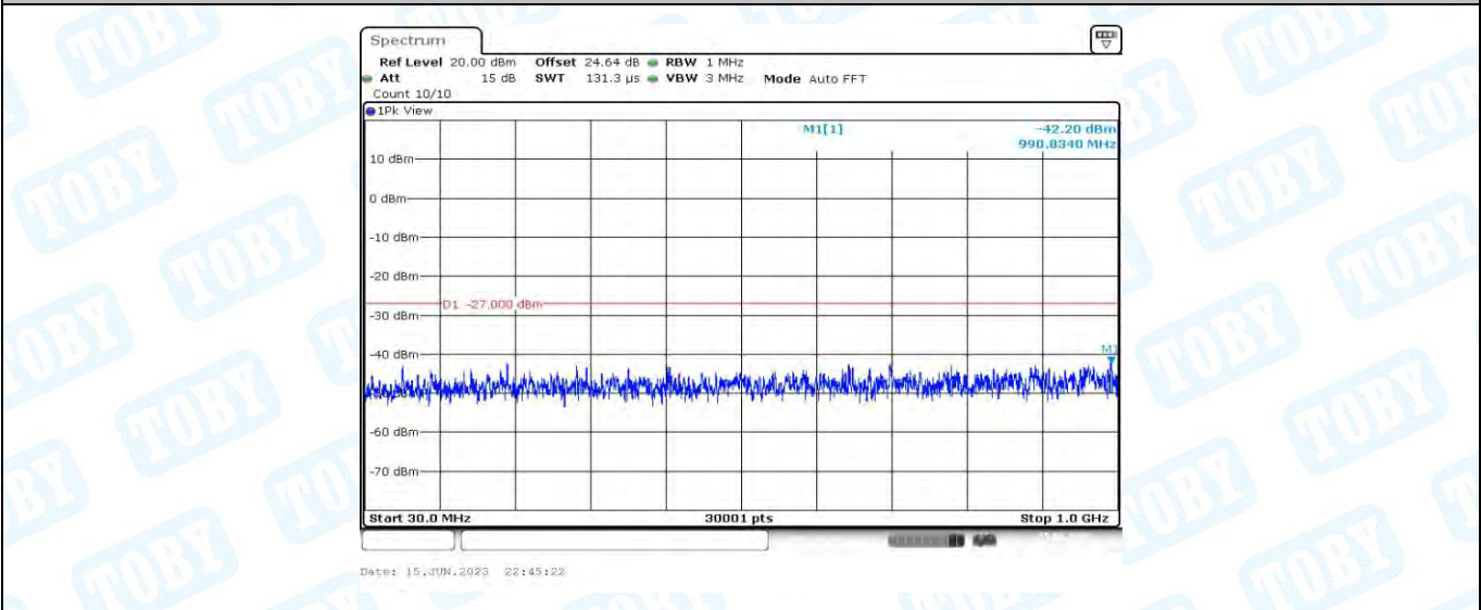
11AX20MIMO_Ant1_5320_30~1000
