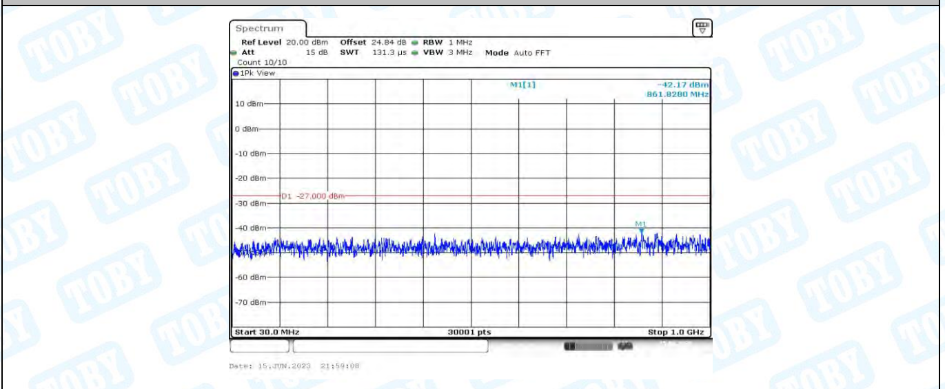
11AC20MIMO_Ant2_5260_30~1000
