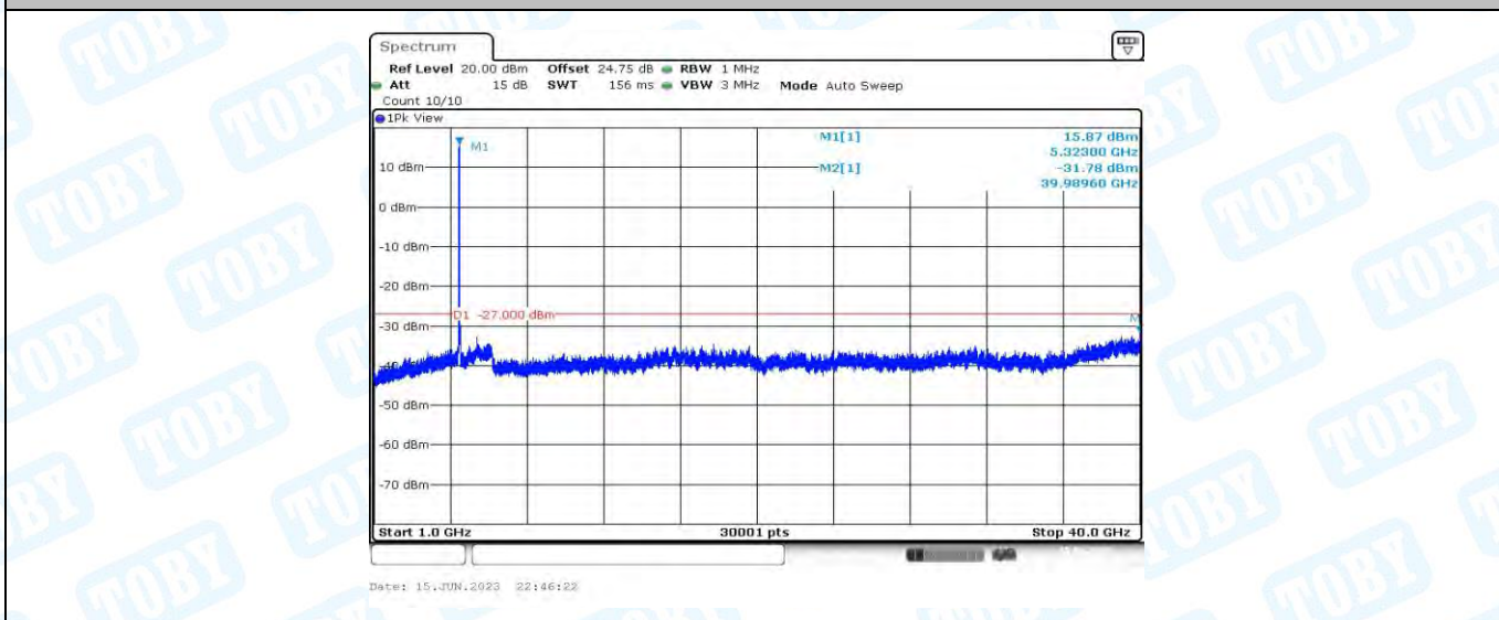
11AX20MIMO_Ant2_5320_1000~40000
