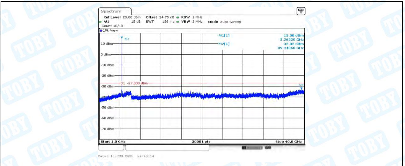
11AX20MIMO_Ant1_5260_1000~40000
