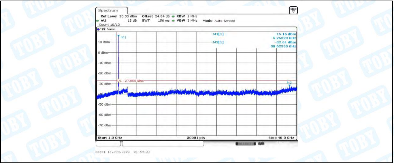
11AC20MIMO_Ant2_5260_1000~40000
