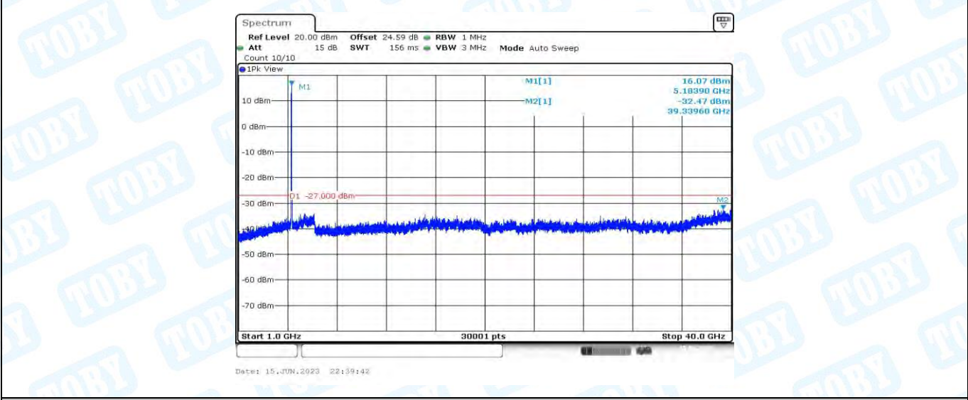
11AX20MIMO_Ant2_5180_1000~40000
