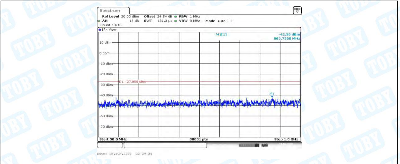
11AC80MIMO_Ant1_5210_30~1000
