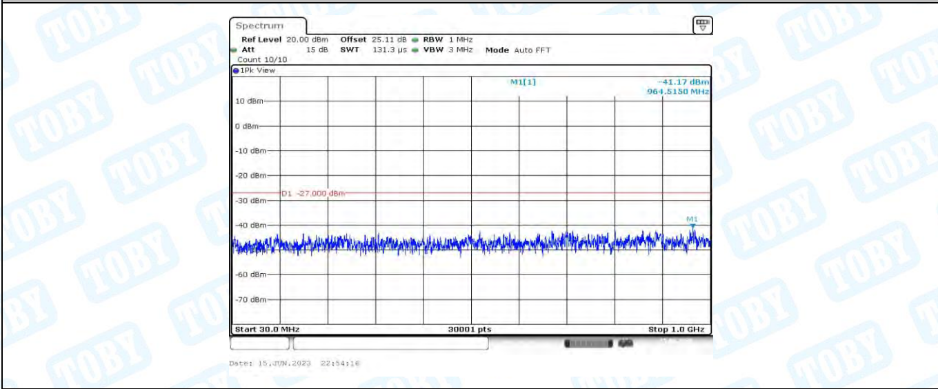
11AX20MIMO_Ant2_5745_30~1000
