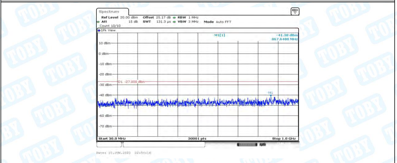
11AX20MIMO_Ant2_5500_30~1000
