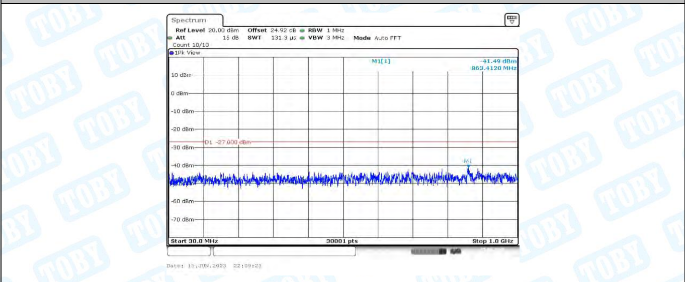
11AC20MIMO_Ant1_5785_30~1000
