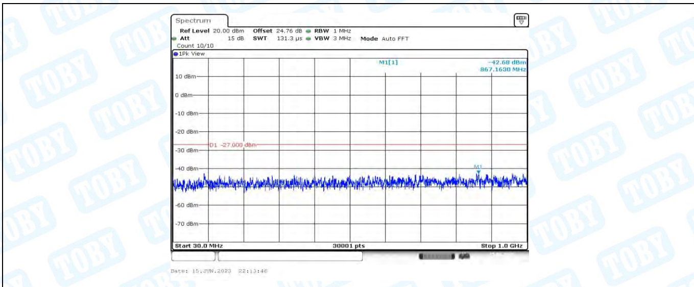
11AC40MIMO_Ant2_5230_30~1000
