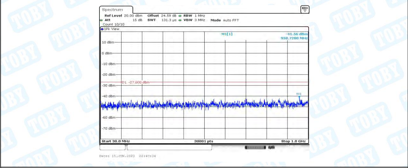
11AX20MIMO_Ant2_5200_30~1000
