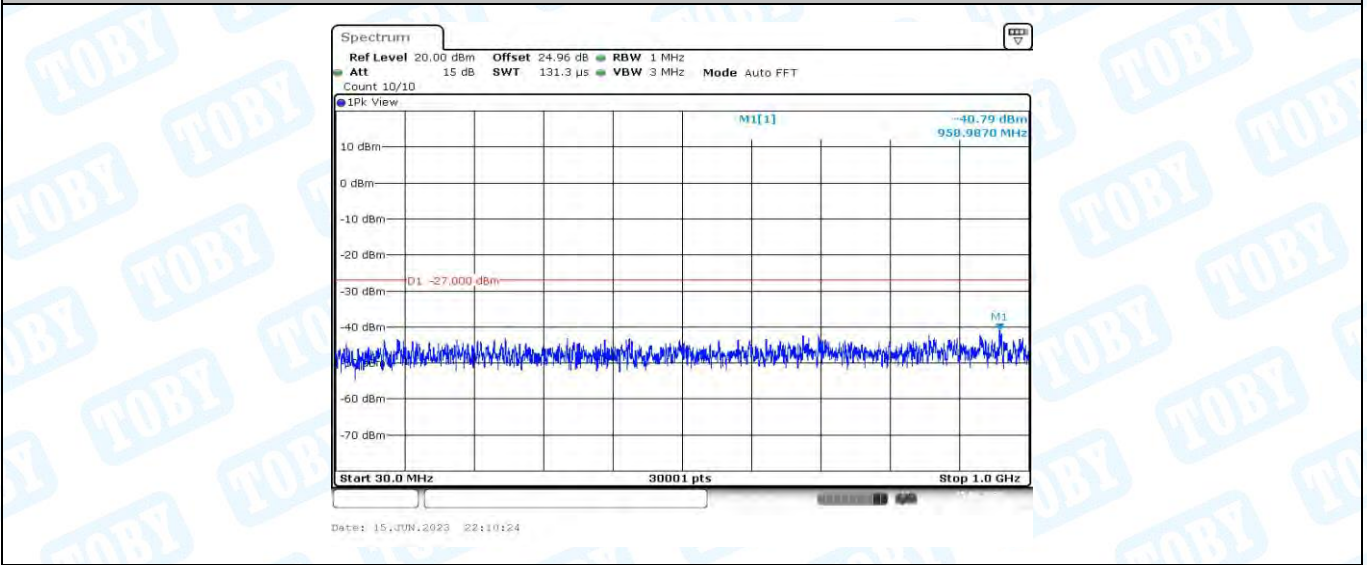
11AC20MIMO_Ant1_5825_30~1000
