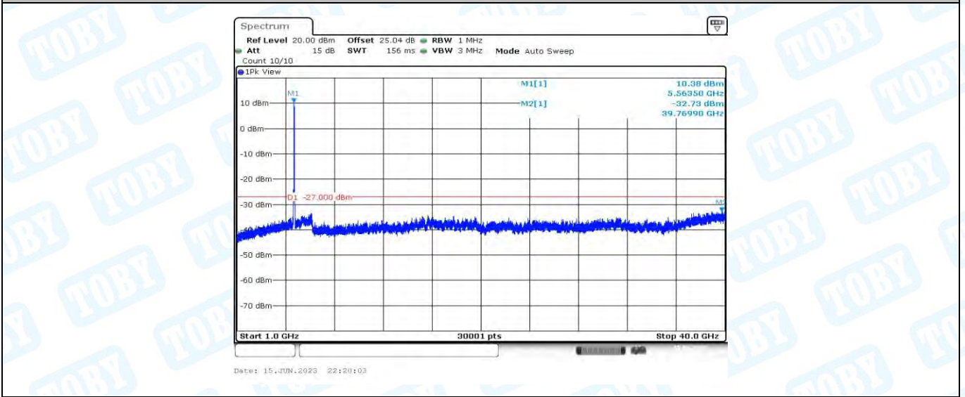
11AC40MIMO_Ant2_5550_1000~40000
