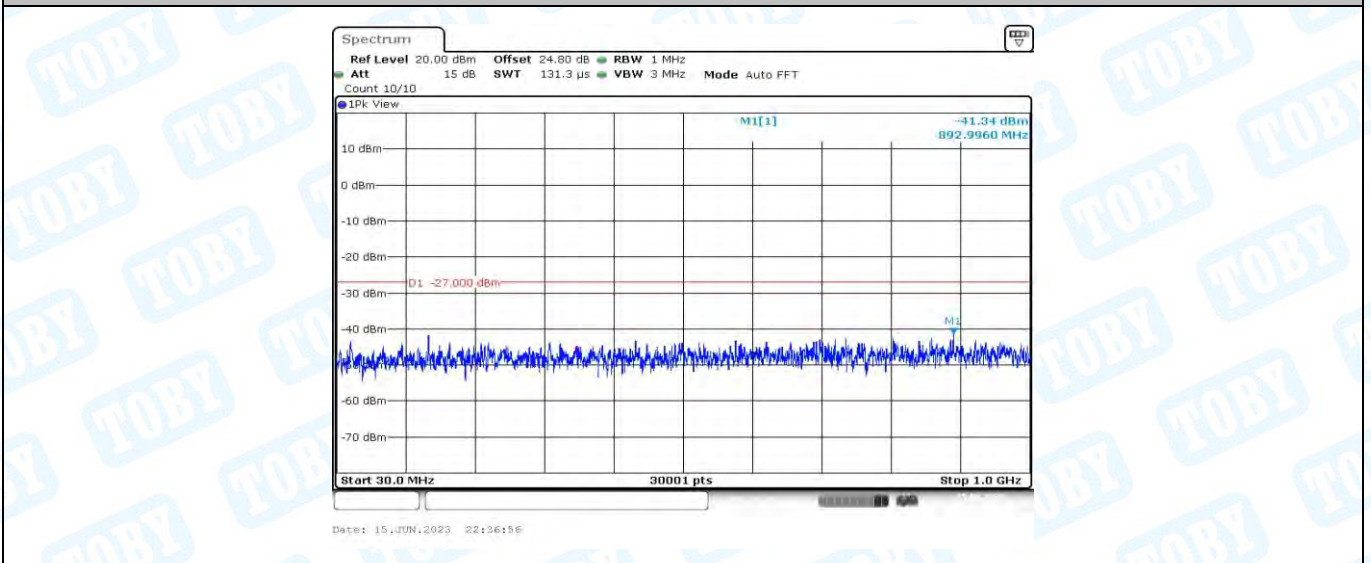
11AC80MIMO_Ant2_5610_30~1000
