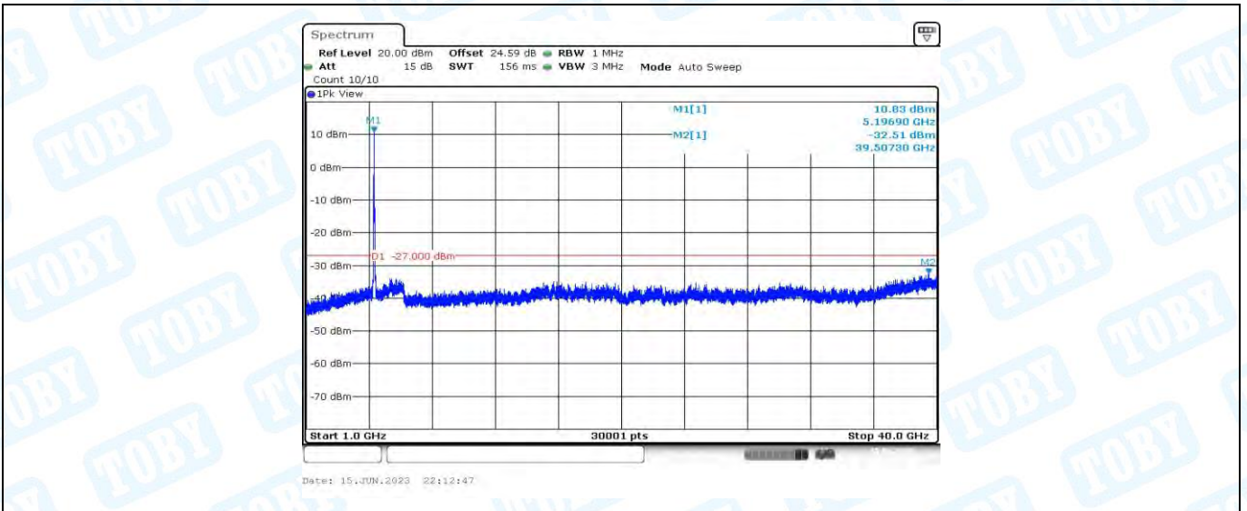
11AC40MIMO_Ant2_5190_1000~40000
