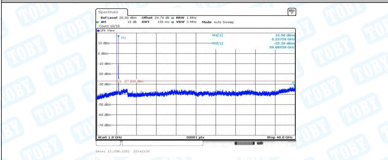
11AX20MIMO_Ant2_5240_1000~40000
