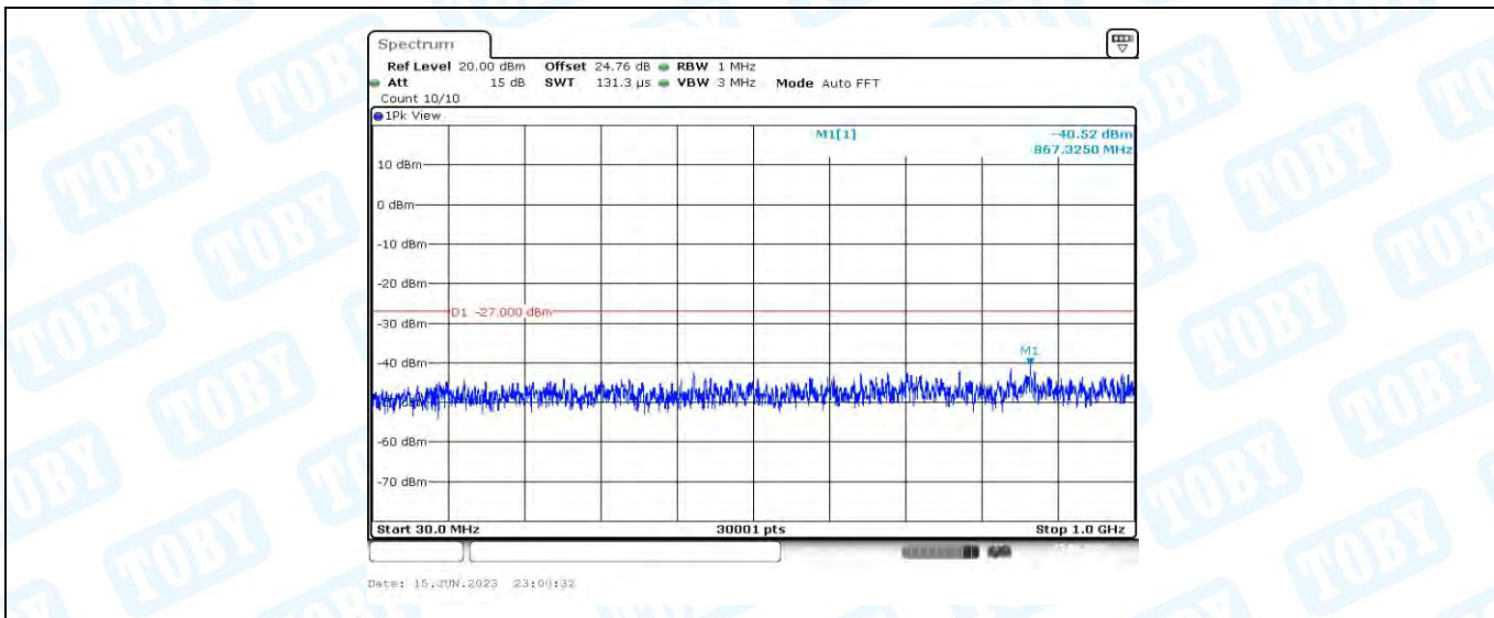
11AX40MIMO_Ant2_5270_30~1000
