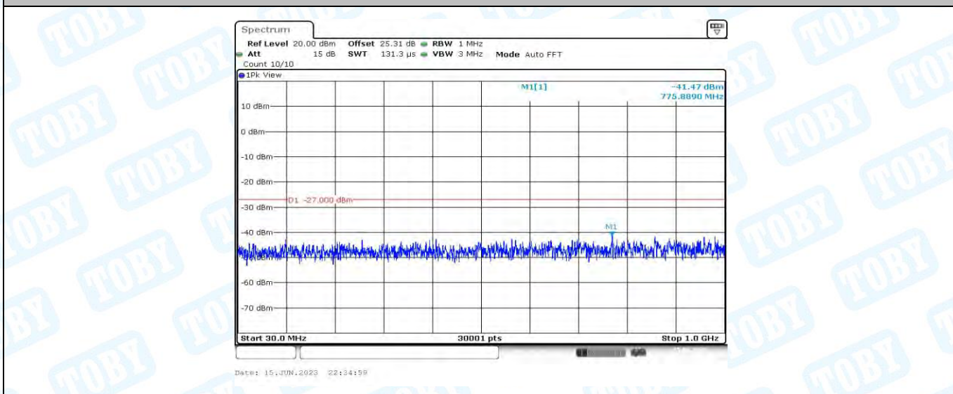
11AC80MIMO_Ant2_5530_30~1000
