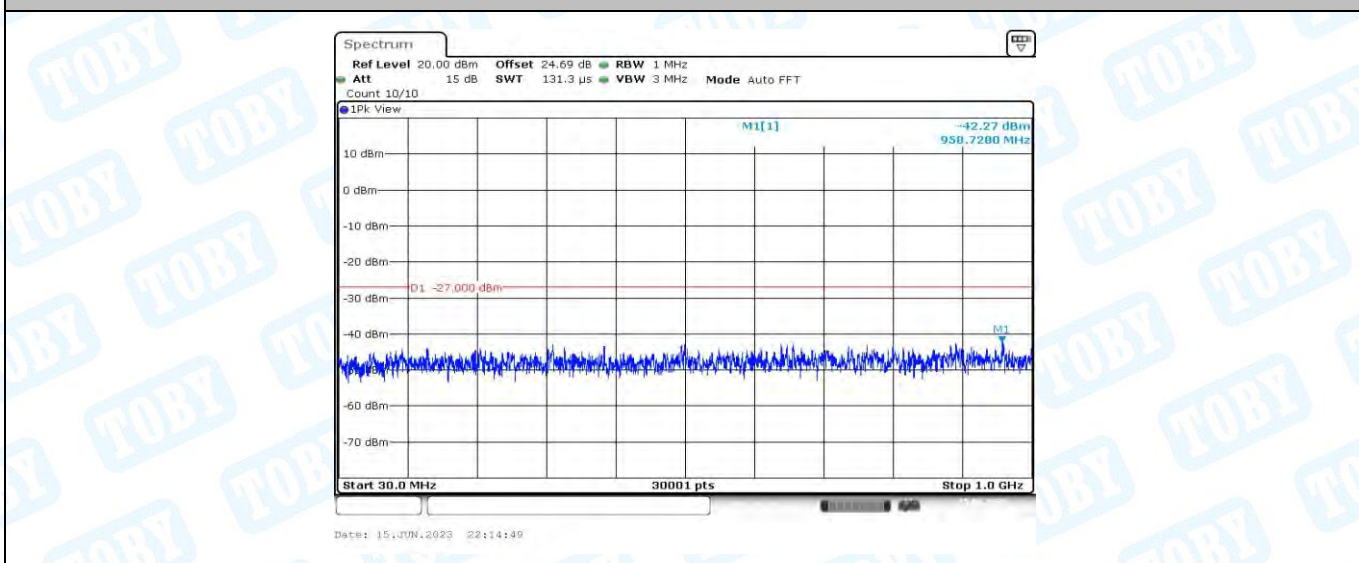
11AC40MIMO_Ant1_5270_30~1000
