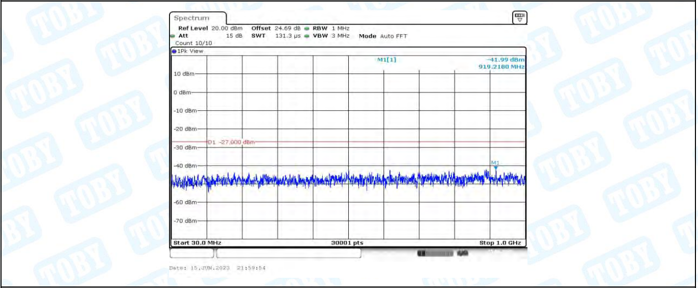
11AC20MIMO_Ant1_5280_30~1000
