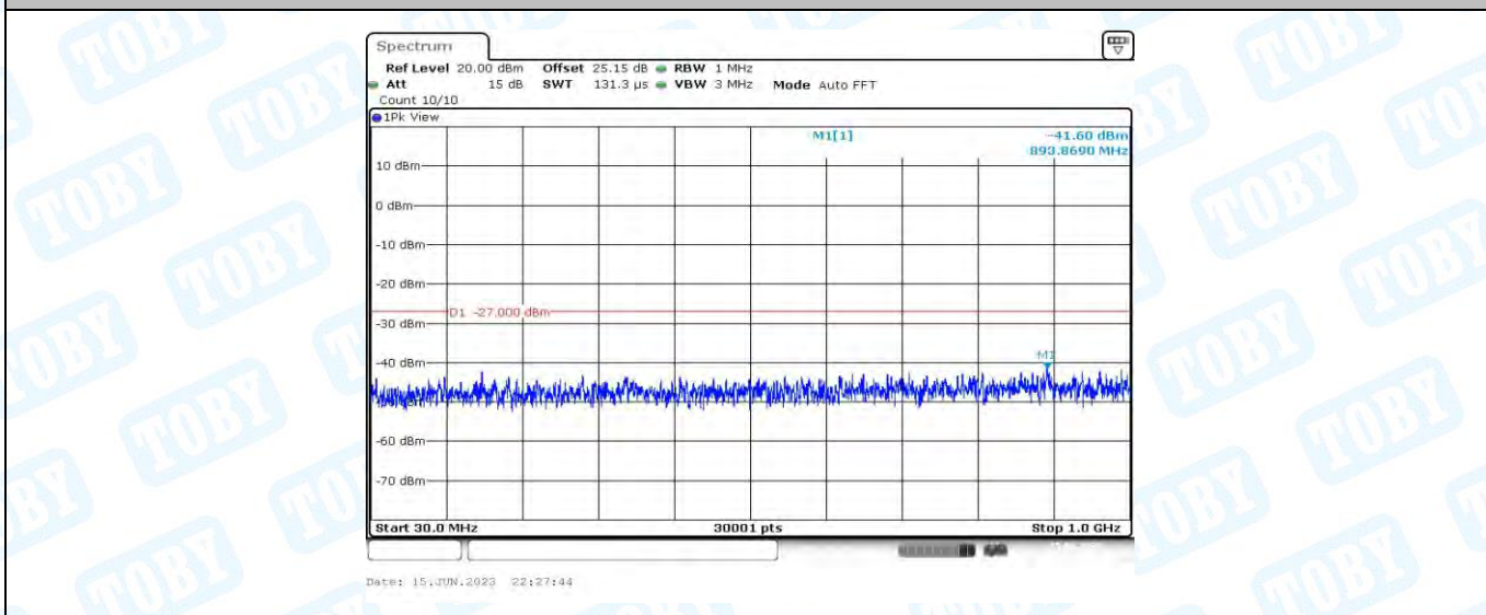
11AC40MIMO_Ant1_5755_30~1000
