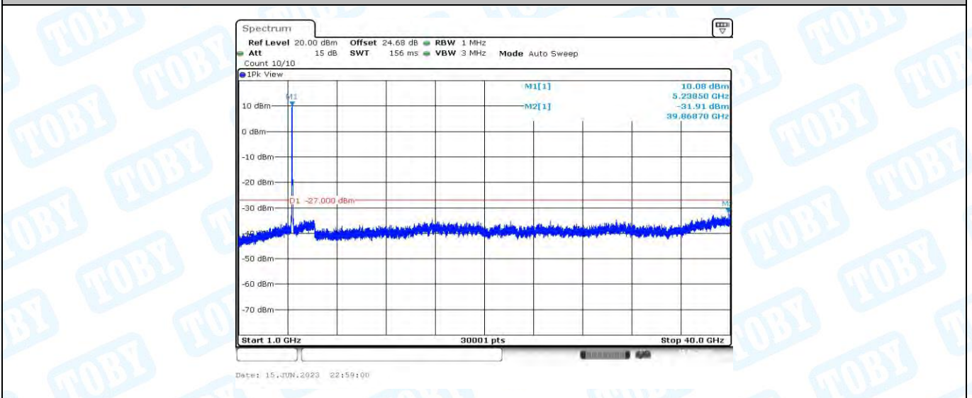
11AX40MIMO_Ant1_5230_1000~40000
