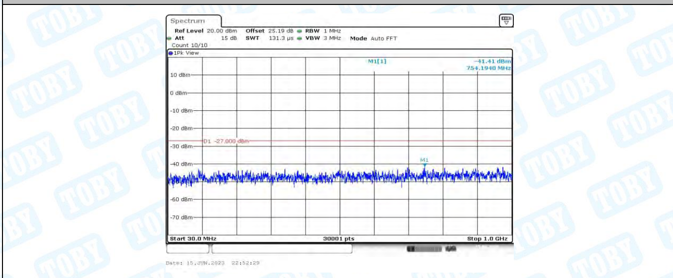
11AX20MIMO_Ant1_5700_30~1000
