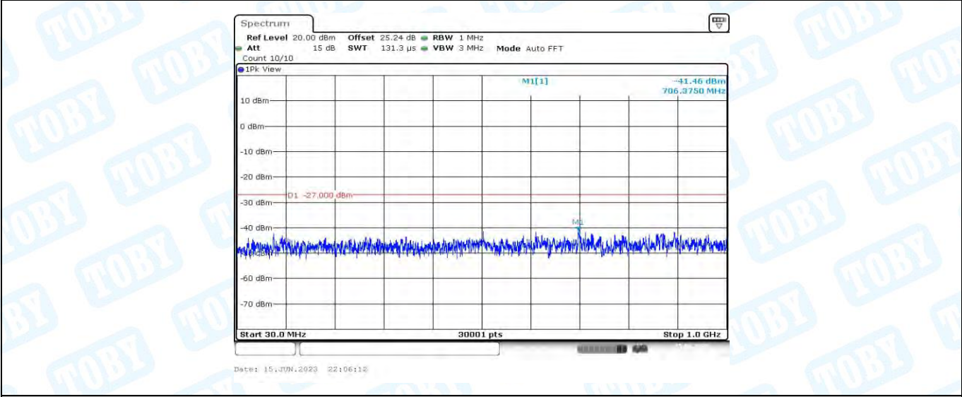
11AC20MIMO_Ant2_5700_30~1000
