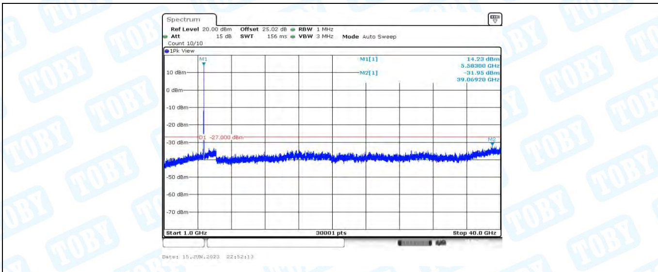
11AX20MIMO_Ant2_5580_1000~40000
