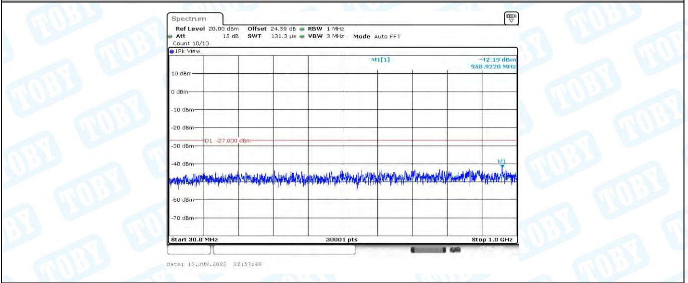
11AX40MIMO_Ant2_5190_30~1000
