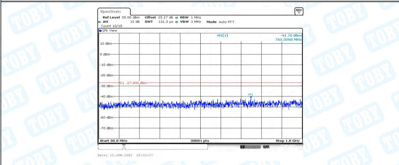
11AC20MIMO_Ant2_5500_30~1000
