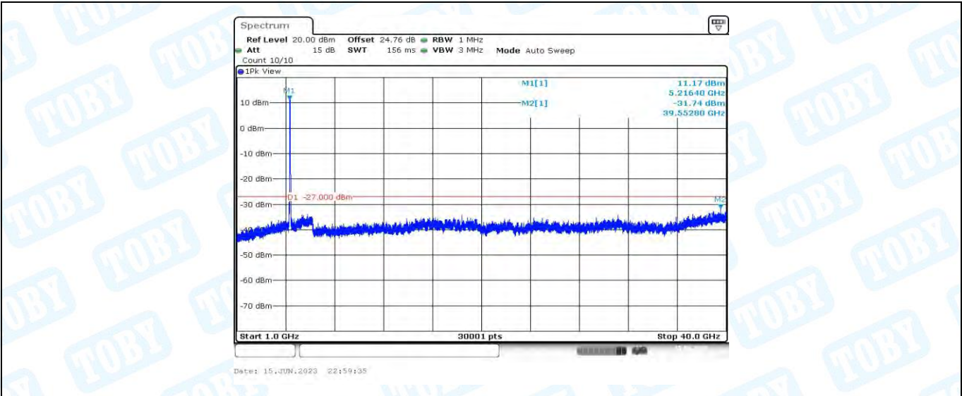
11AX40MIMO_Ant2_5230_1000~40000
