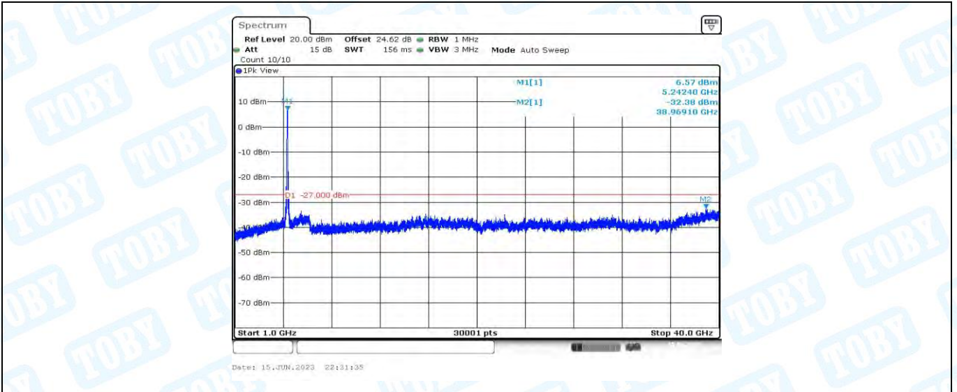
11AC80MIMO_Ant2_5210_1000~40000
