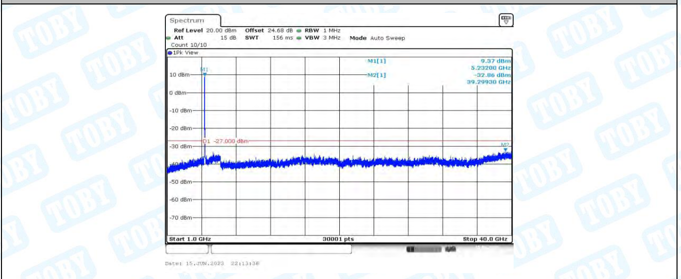
11AC40MIMO_Ant1_5230_1000~40000
