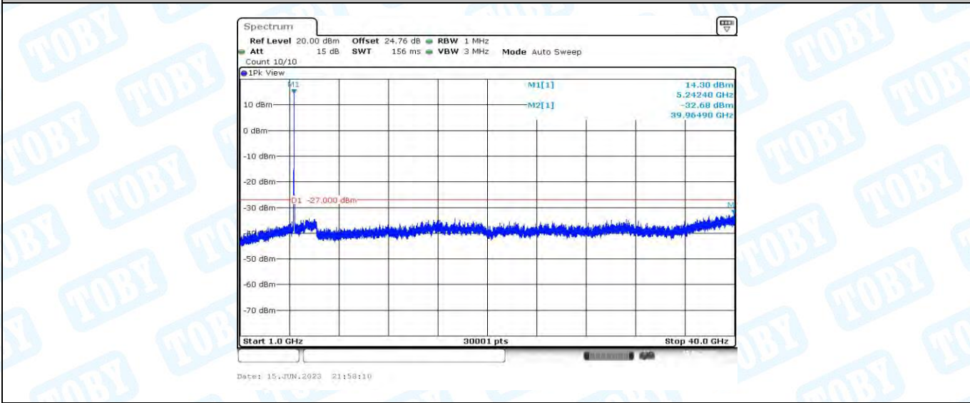
11AC20MIMO_Ant2_5240_1000~40000
