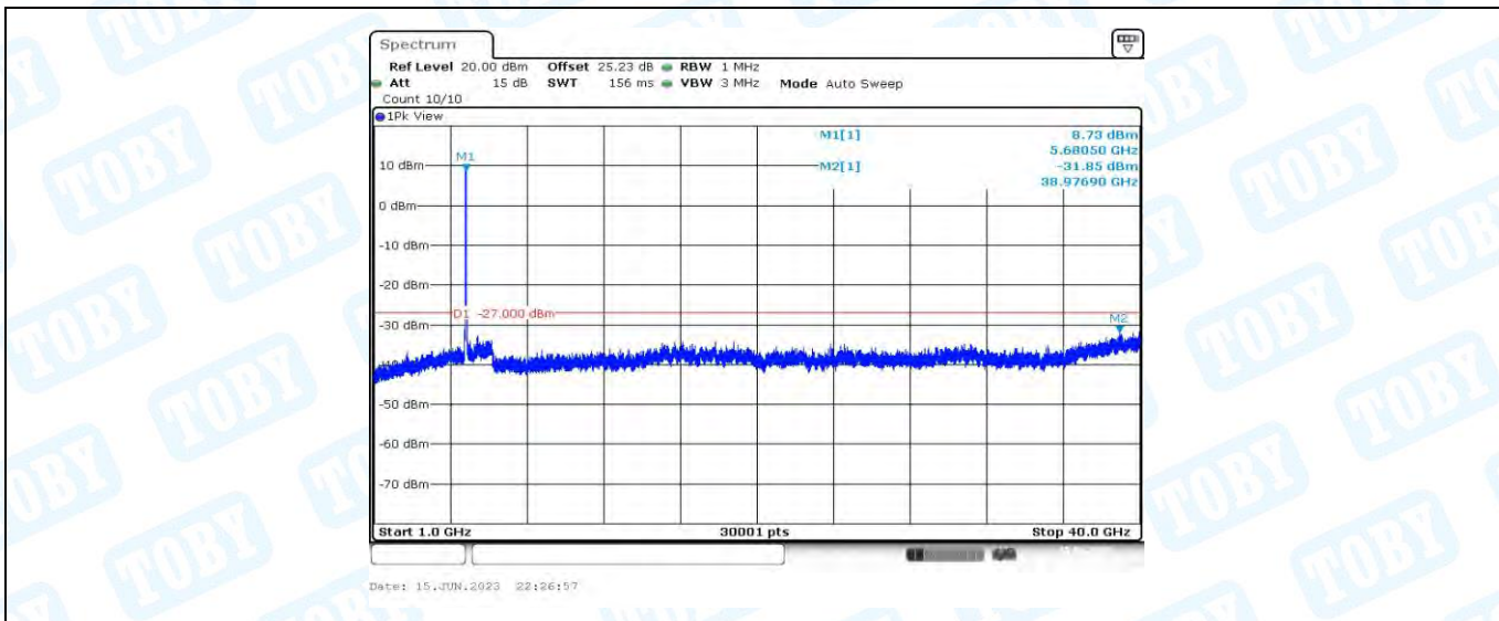
11AC40MIMO_Ant2_5670_1000~40000
