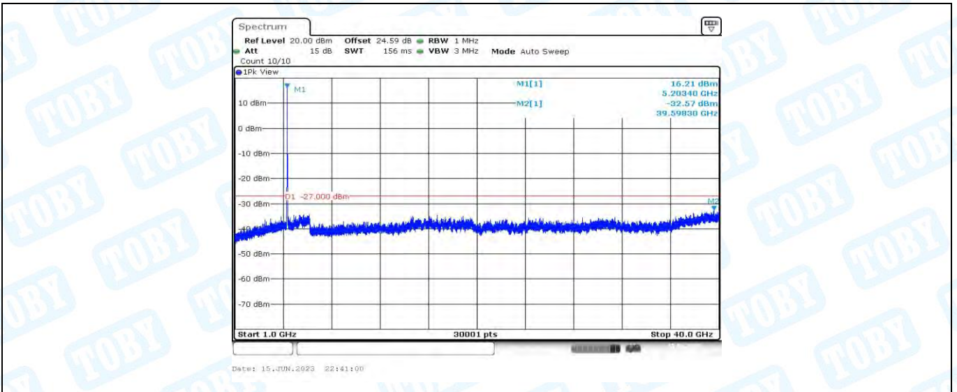
11AX20MIMO_Ant2_5200_1000~40000
