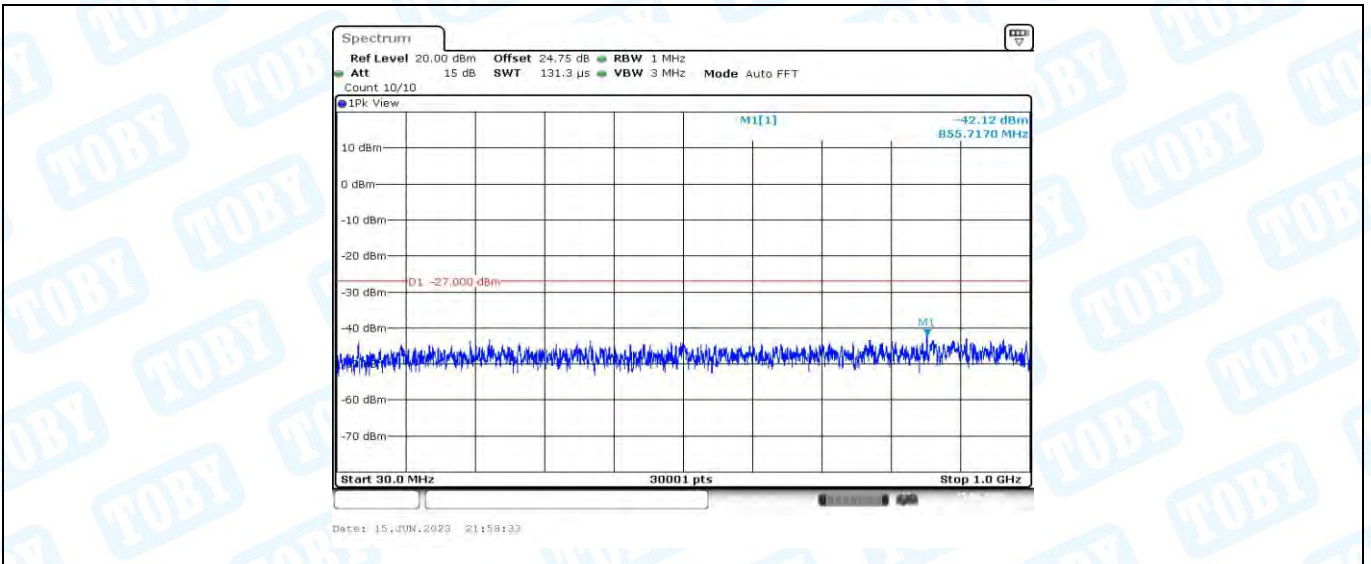
11AC20MIMO_Ant1_5260_30~1000
