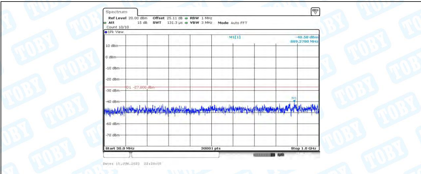
11AC40MIMO_Ant2_5755_30~1000
