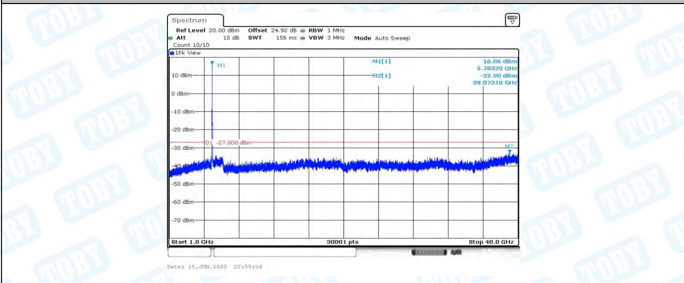
11AX20MIMO_Ant1_5785_1000~40000
