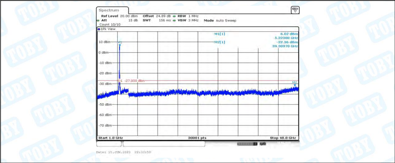
11AC80MIMO_Ant2_5290_1000~40000
