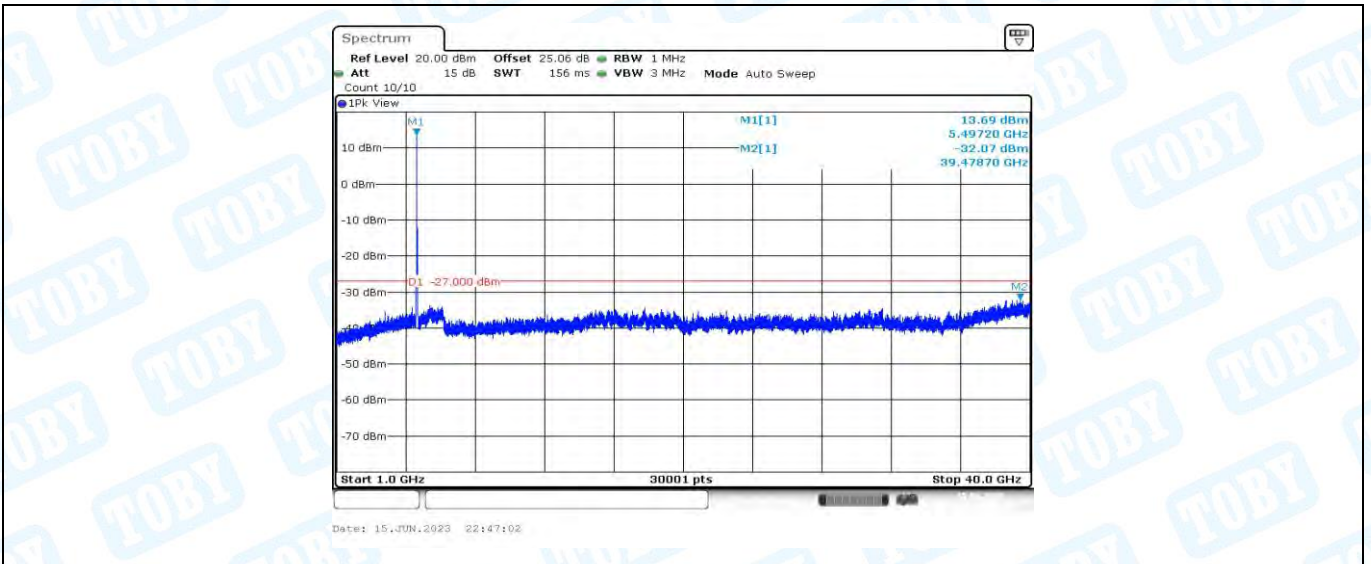
11AX20MIMO_Ant1_5500_1000~40000
