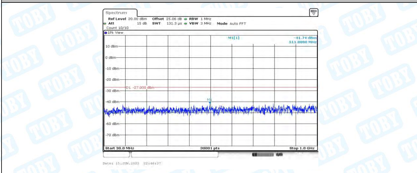
11AX20MIMO_Ant1_5500_30~1000
