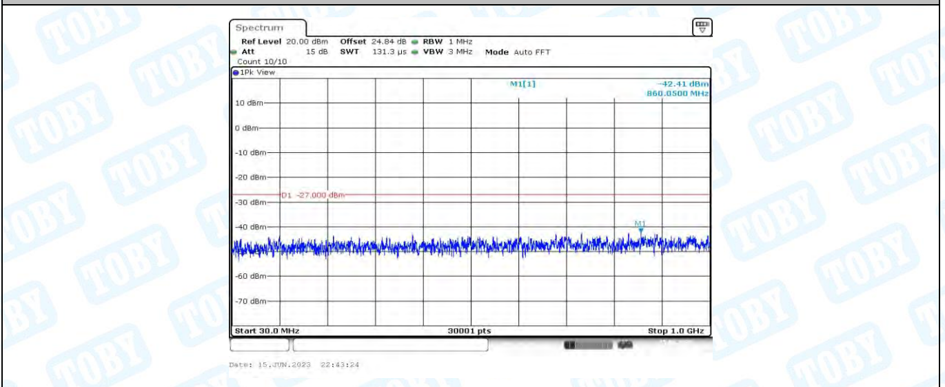
11AX20MIMO_Ant2_5260_30~1000
