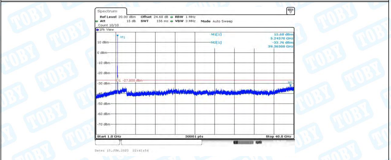
11AX20MIMO_Ant1_5240_1000~40000
