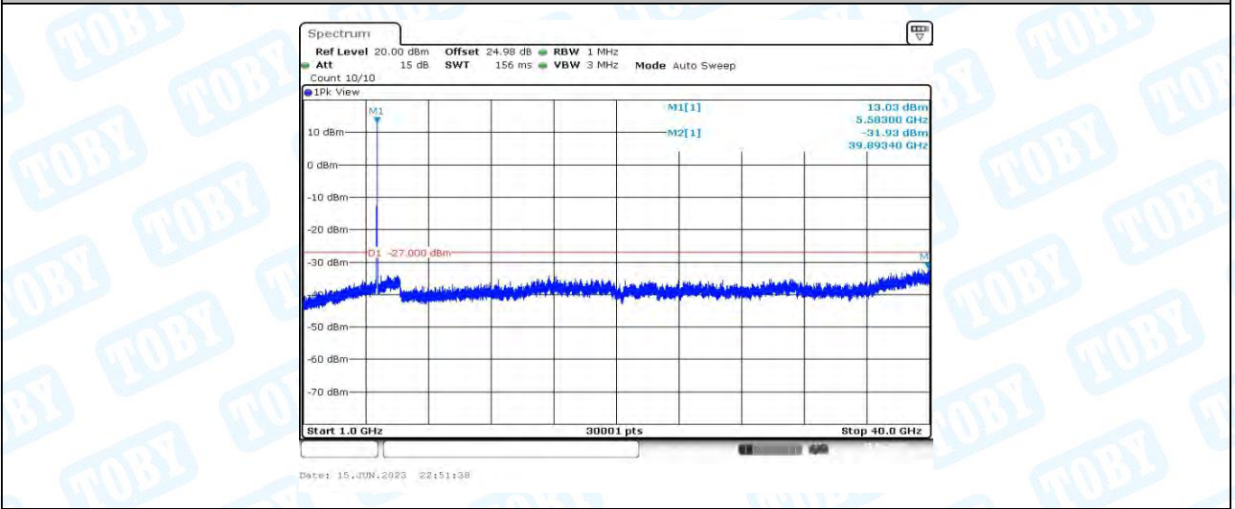
11AX20MIMO_Ant1_5580_1000~40000
