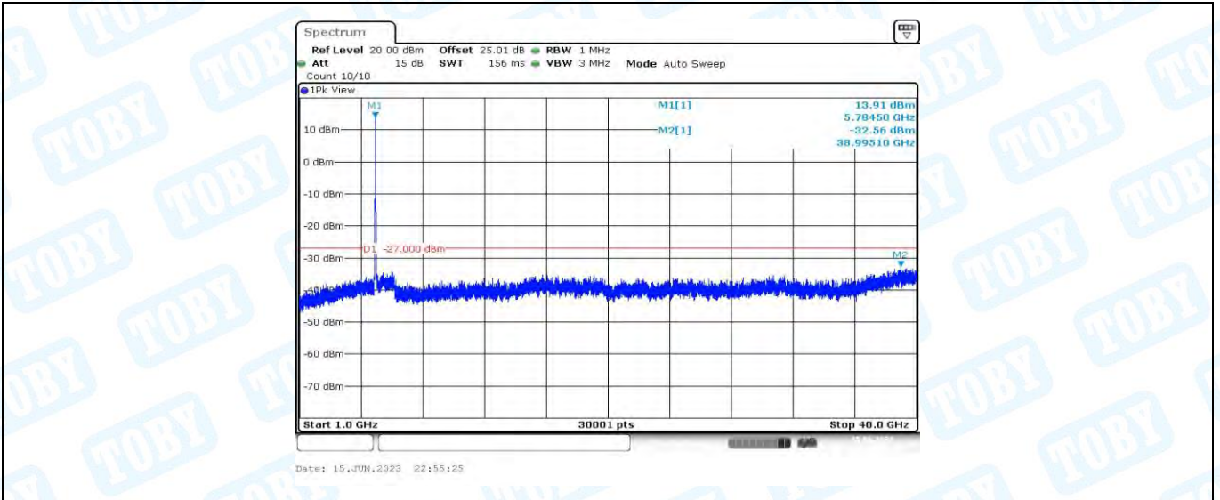
11AX20MIMO_Ant2_5785_1000~40000
