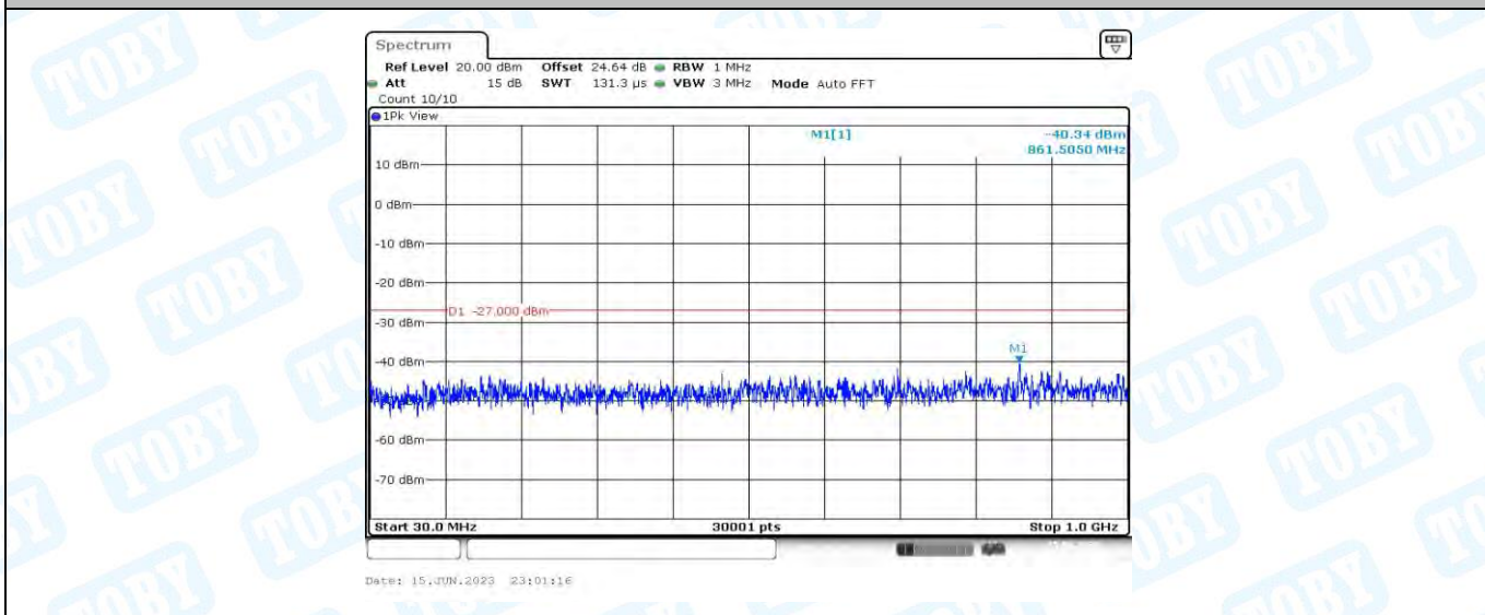
11AX40MIMO_Ant1_5310_30~1000
