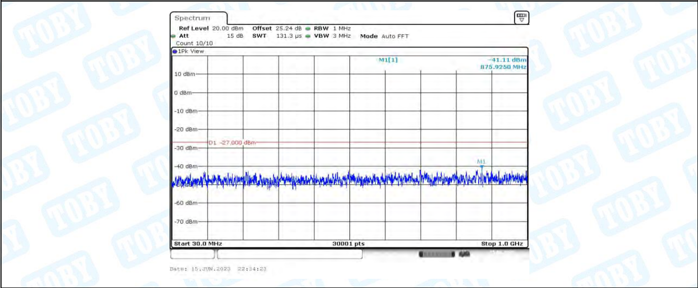
11AC80MIMO_Ant1_5530_30~1000
