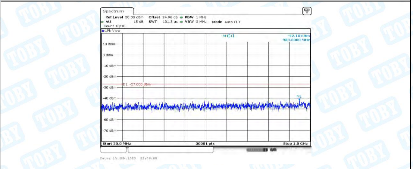
11AX20MIMO_Ant1_5825_30~1000
