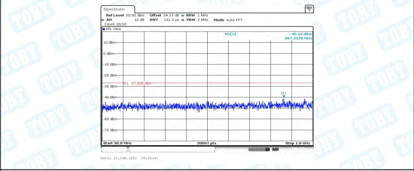
11AX20MIMO_Ant1_5180_30~1000
