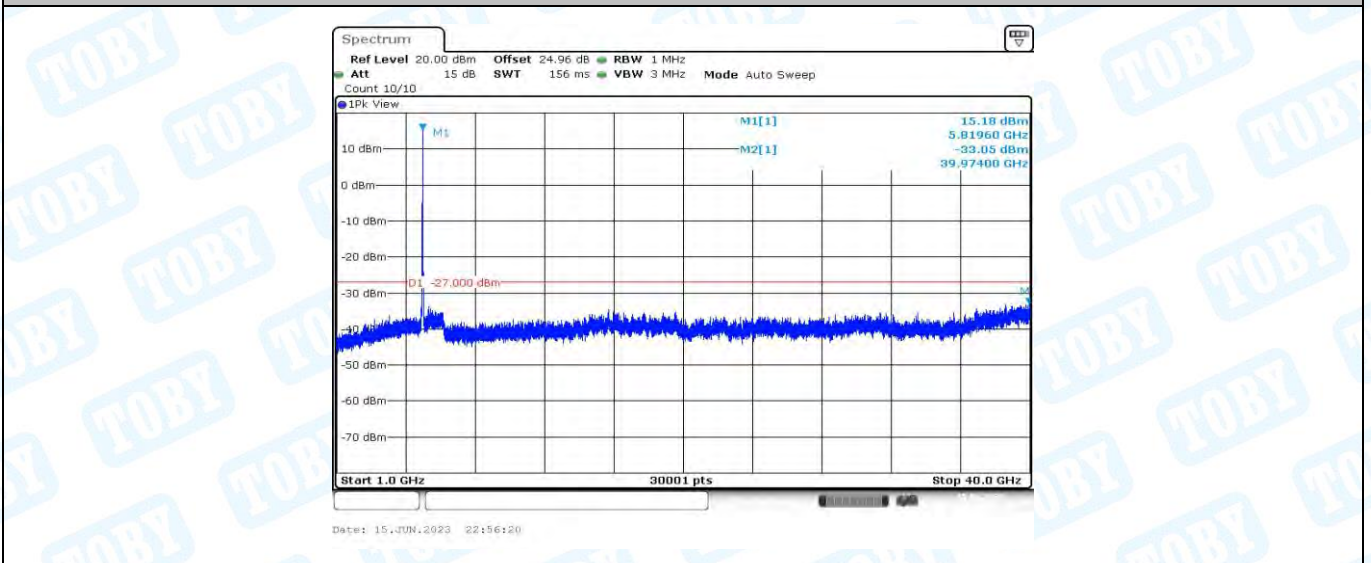
11AX20MIMO_Ant1_5825_1000~40000
