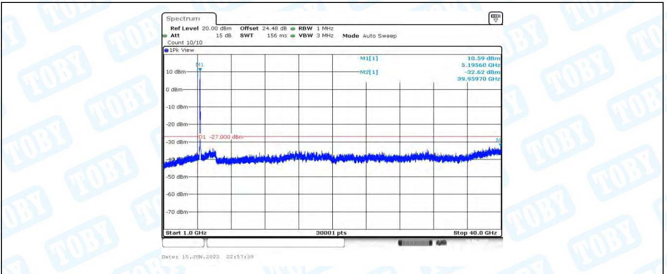
11AX40MIMO_Ant1_5190_1000~40000
