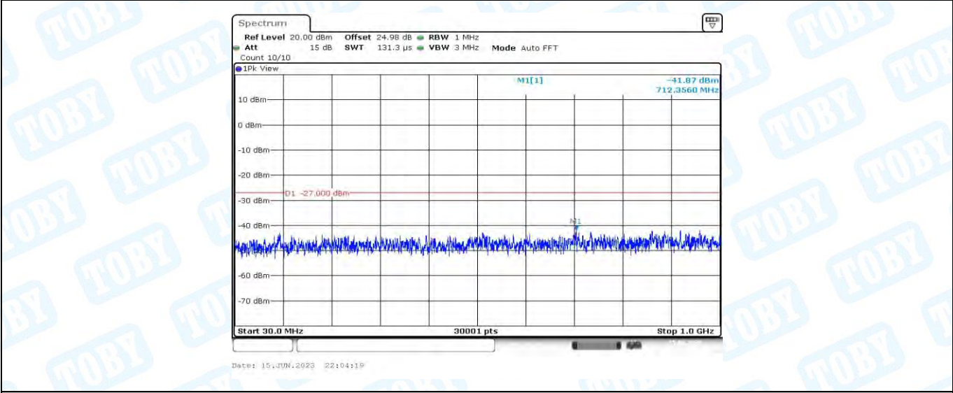
11AC20MIMO_Ant1_5580_30~1000
