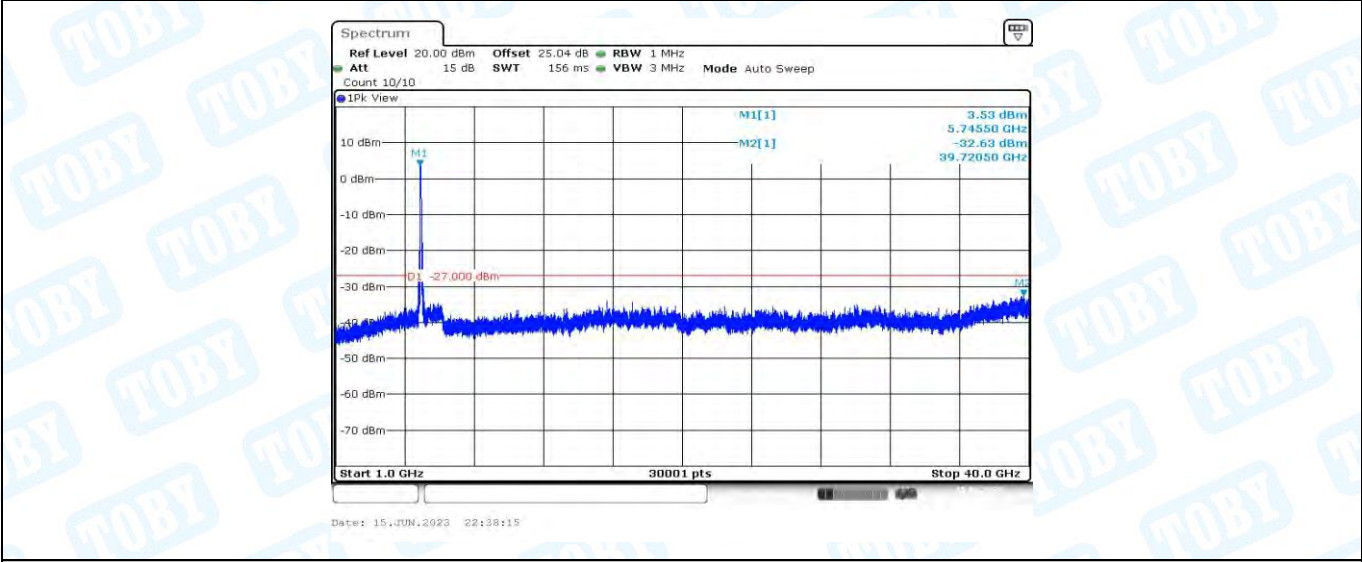
11AC80MIMO_Ant2_5775_1000~40000
