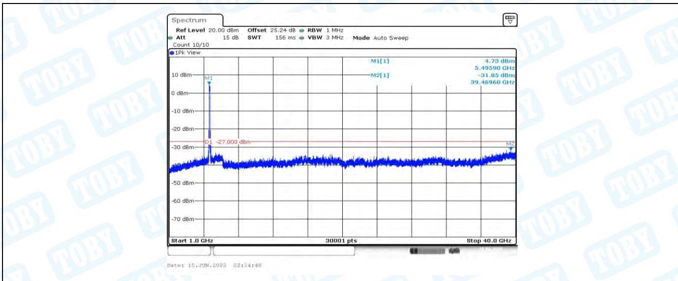
11AC80MIMO_Ant1_5530_1000~40000
