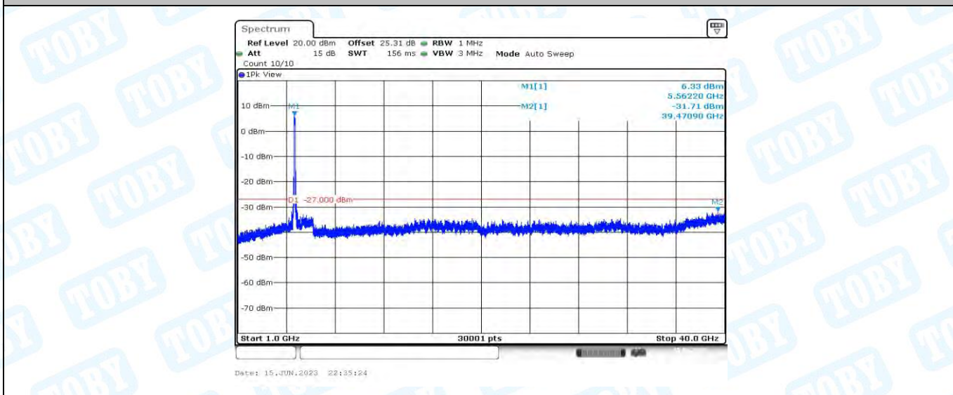
11AC80MIMO_Ant2_5530_1000~40000
