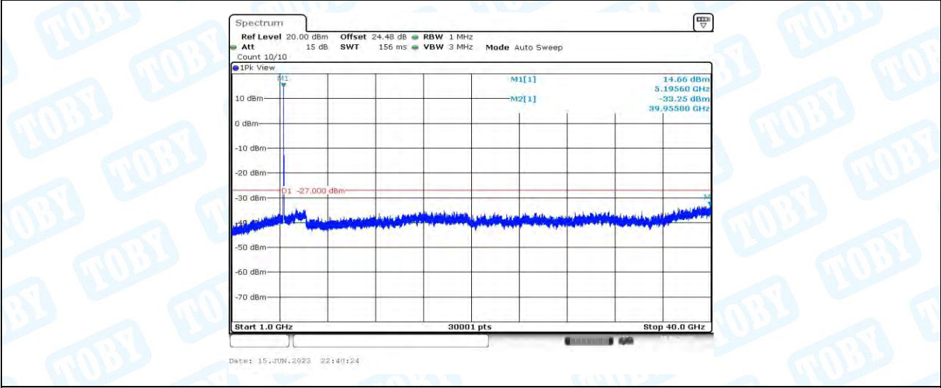
11AX20MIMO_Ant1_5200_1000~40000
