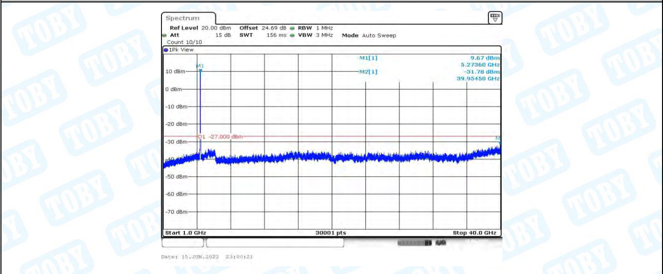
11AX40MIMO_Ant1_5270_1000~40000
