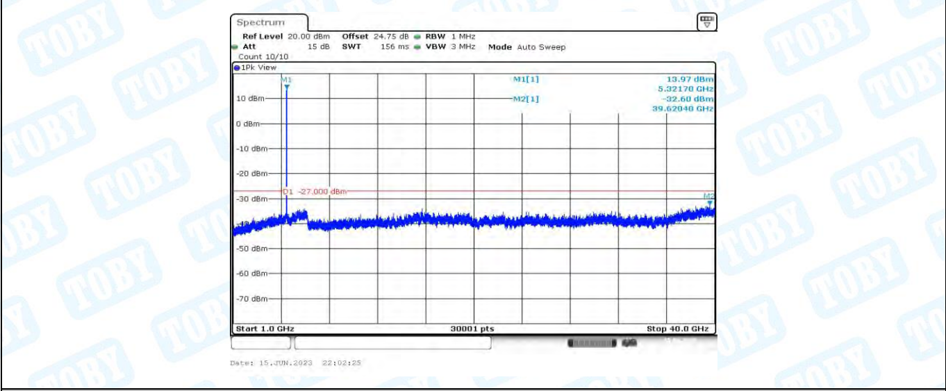
11AC20MIMO_Ant2_5320_1000~40000
