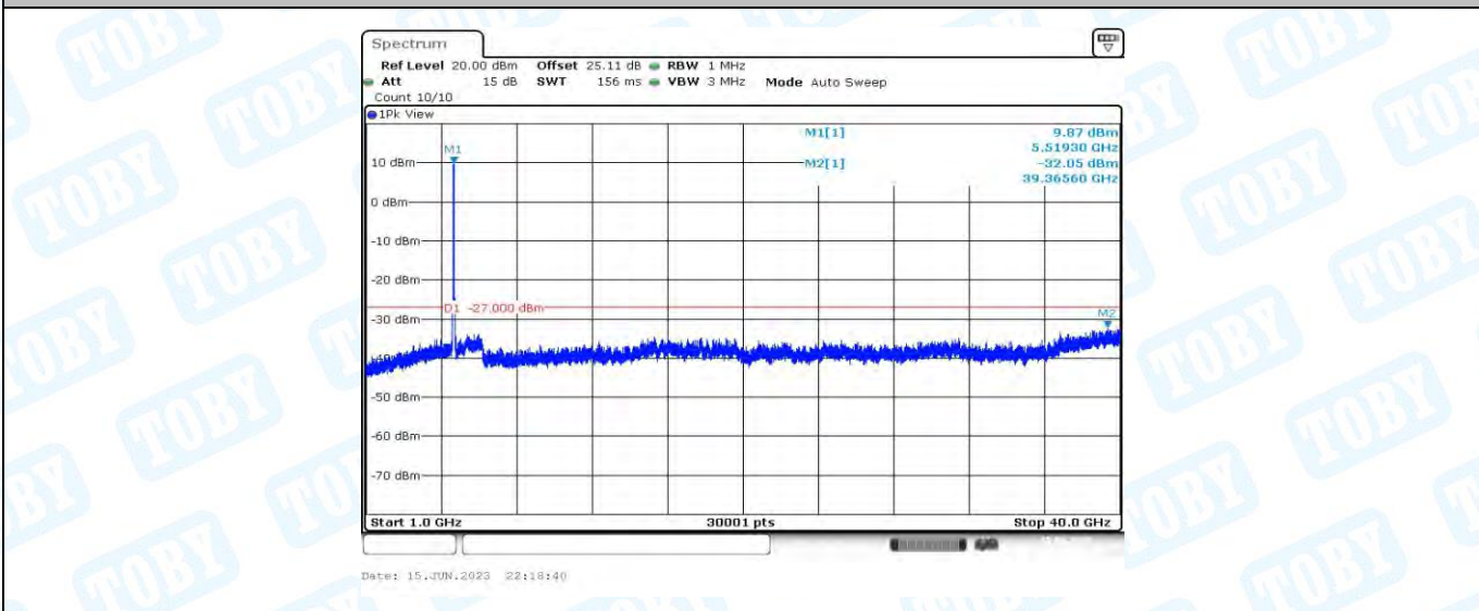
11AC40MIMO_Ant2_5510_1000~40000
