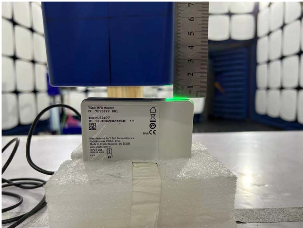
Bottom Side_10mm
