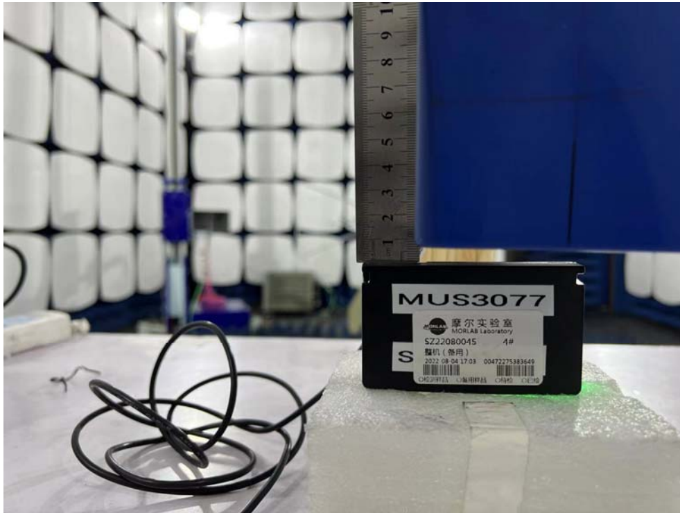
Top Side_10mm
