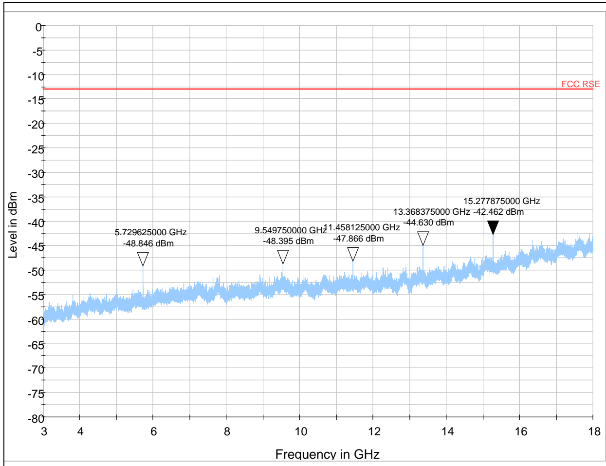
GSM 1900 810 Channel 3GHz ~18GHz
