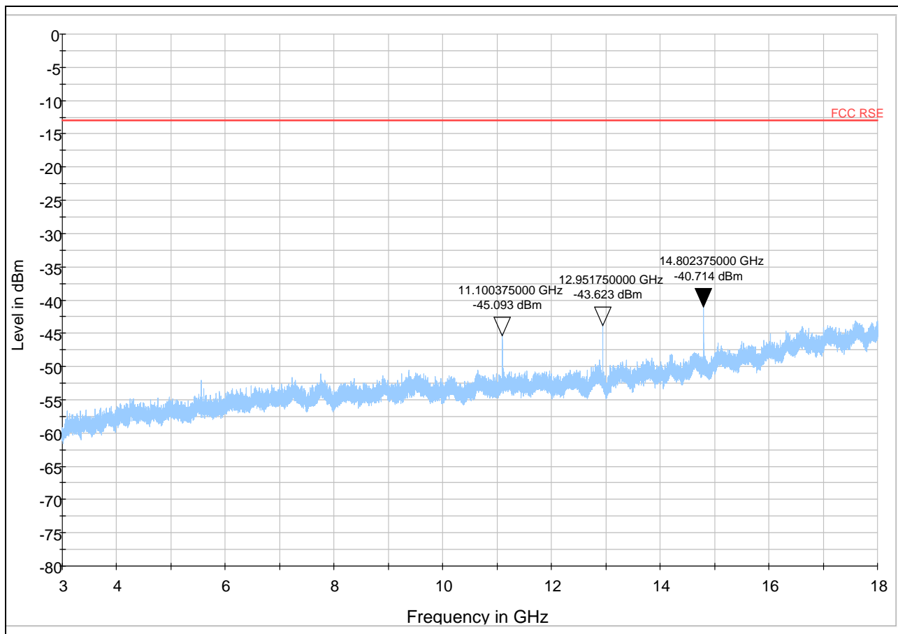
GSM 1900 512 Channel 3GHz ~18GHz
