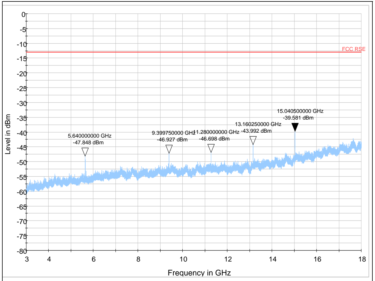
GSM 1900 661 Channel 3GHz ~18GHz
