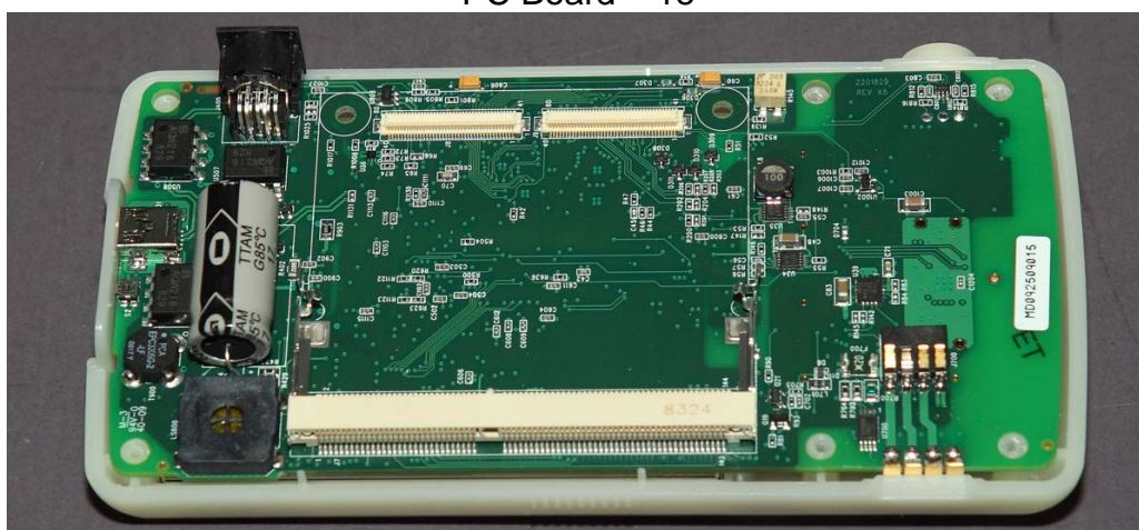
PC Board – 1e
