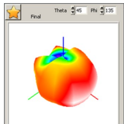
5300MHZ
