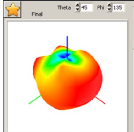
2500MHZ
