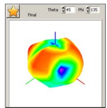
5300MHZ
