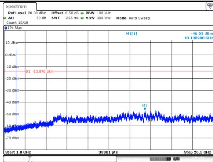
\pi/4 -DQPSK_2441_1000~26500
