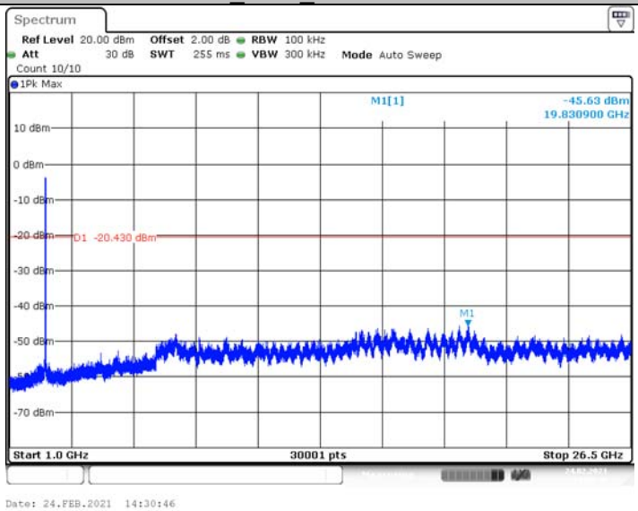
802.11n(HT20) 2412_0~Reference
