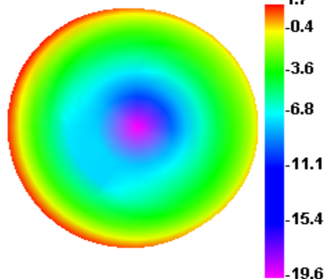
2400.000MHz
