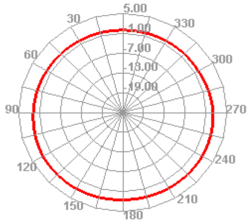
2400.000MHz H
