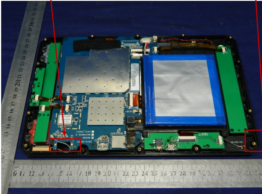
GPS Antenna
