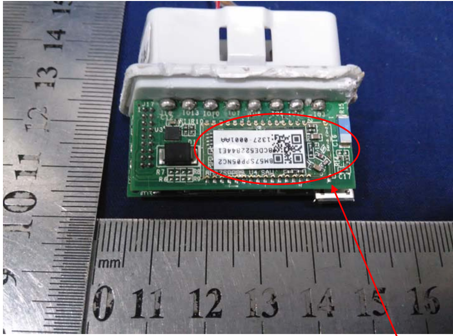
Bluetooth Module
