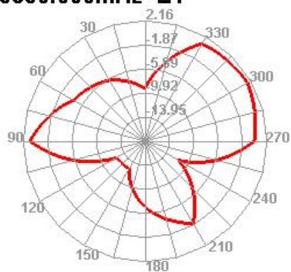
5850.000MHz E1
