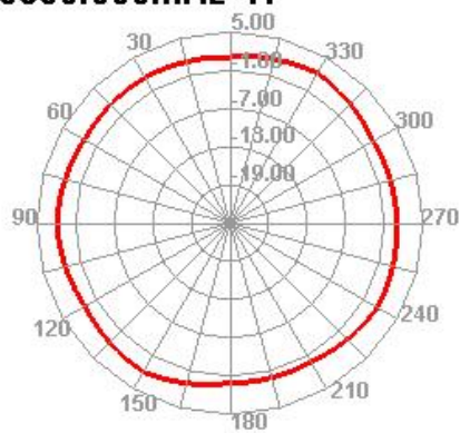
5850.000MHz H
