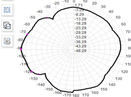
2450.0MHz Total(E2-YZ), Max= 0.98dBi
