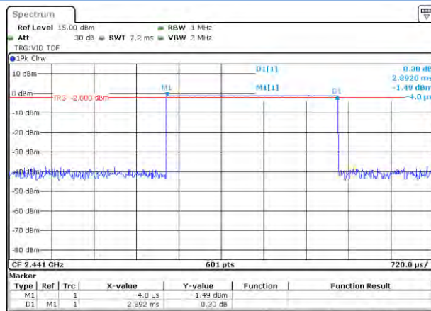
GFSK DH5
