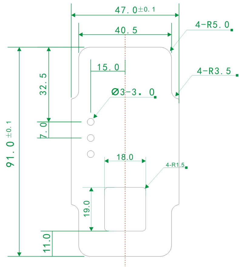
(尺寸图)
