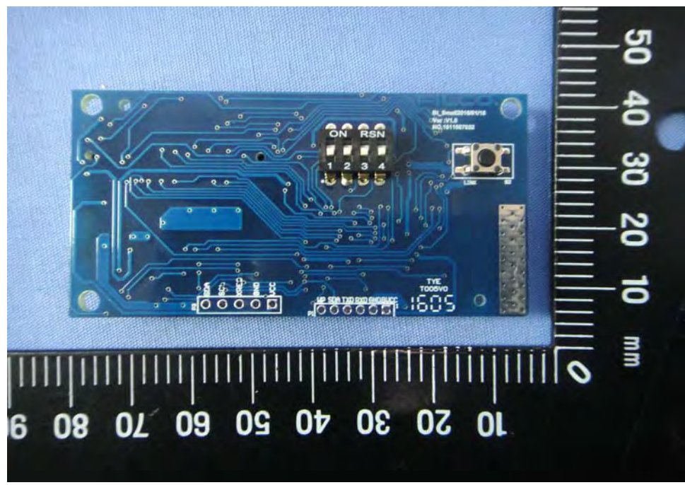
EUT Photo 6 )
