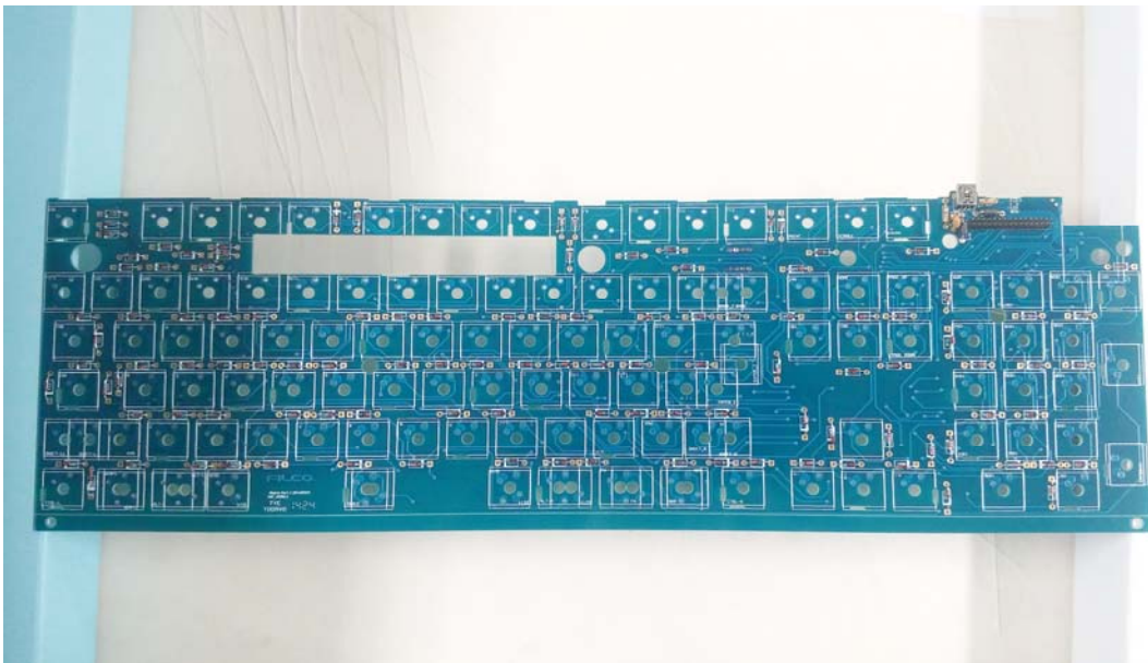
EUT Photo 8 )
