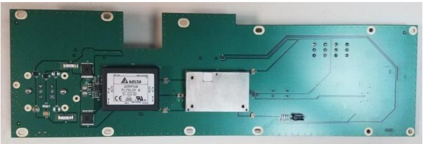
7844370-00 PCBA P4393 WCS-4U DC-DC PSU
