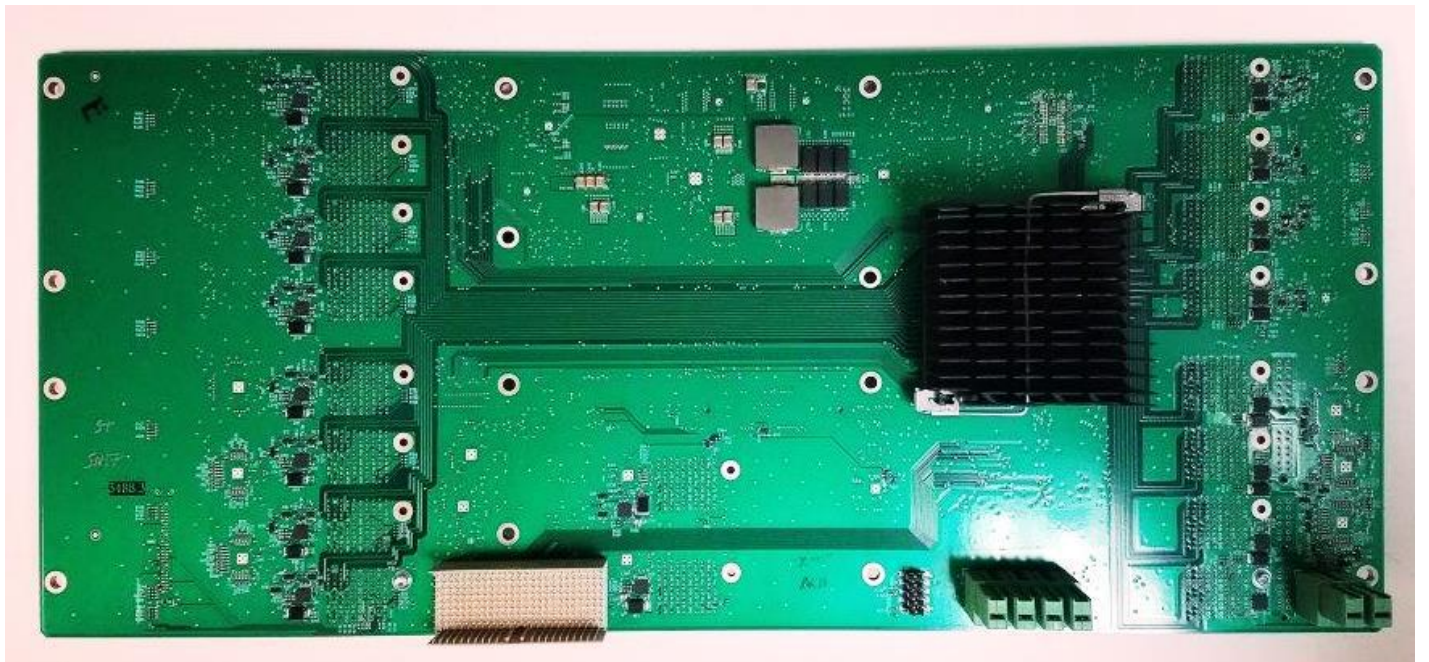
7630167-06 PCB P3488 WCS4 BACKPLANE
