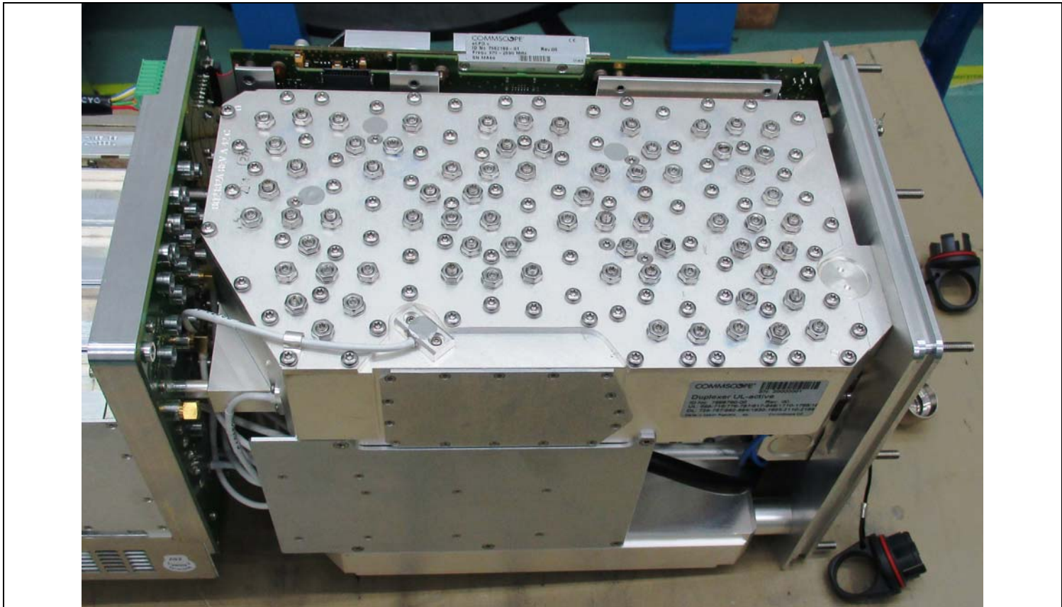
Duplexer
