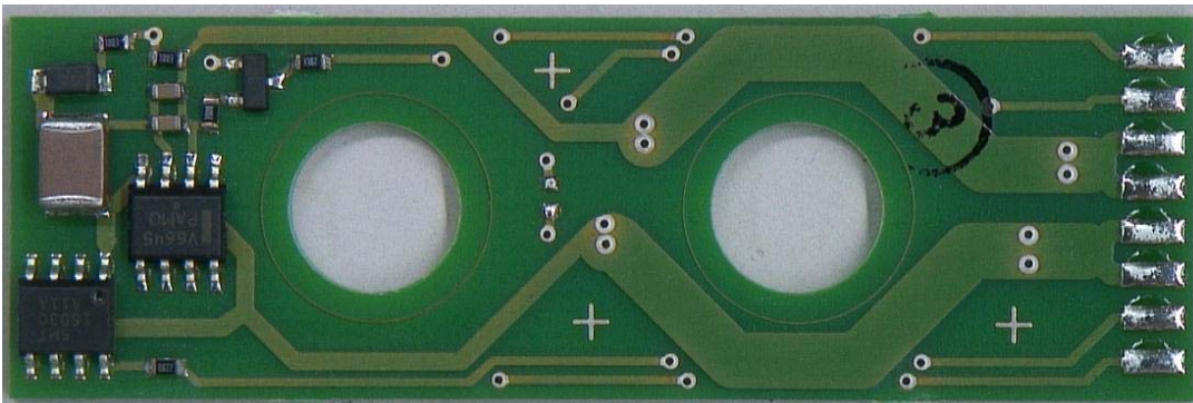
PCB P3683 FanUnitBoard M2-Cab 7659273-00
