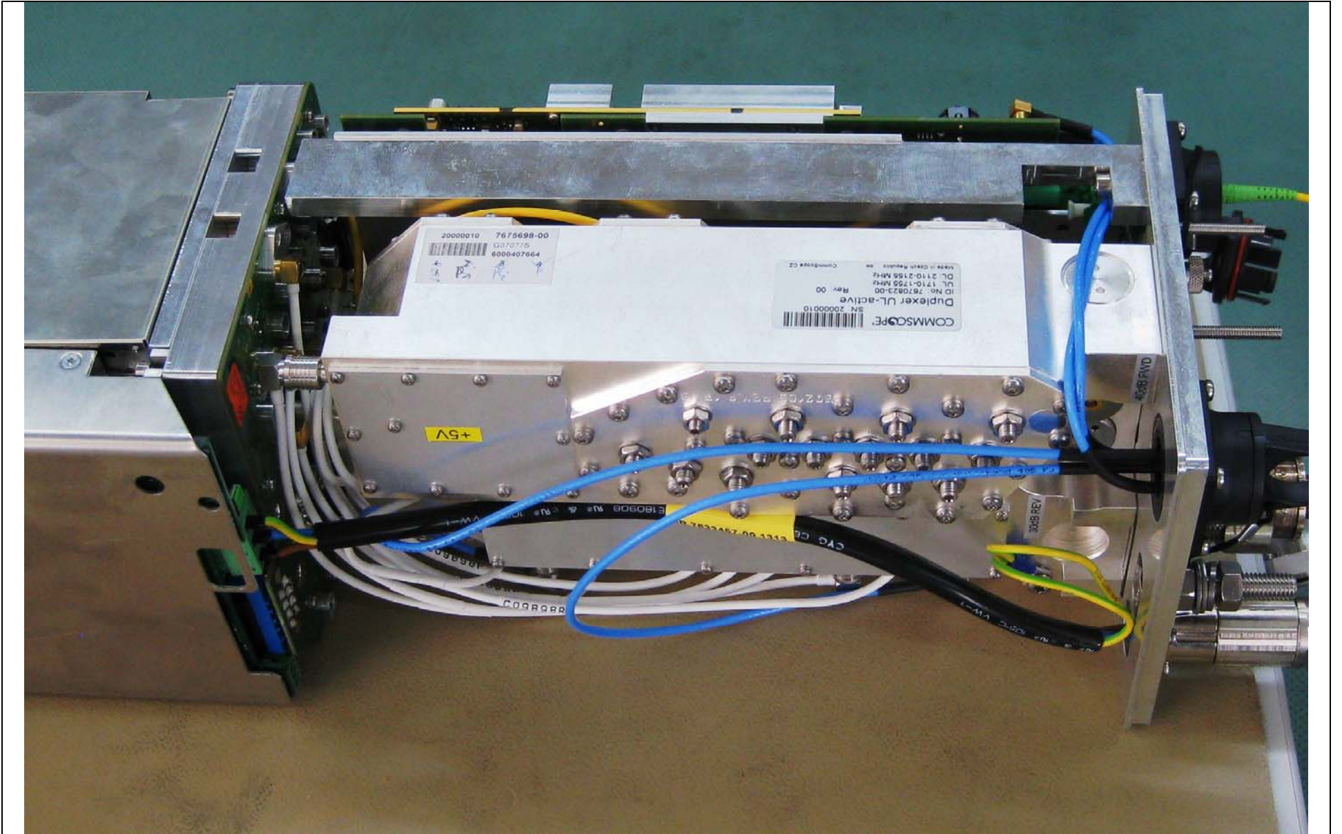
Duplexer
