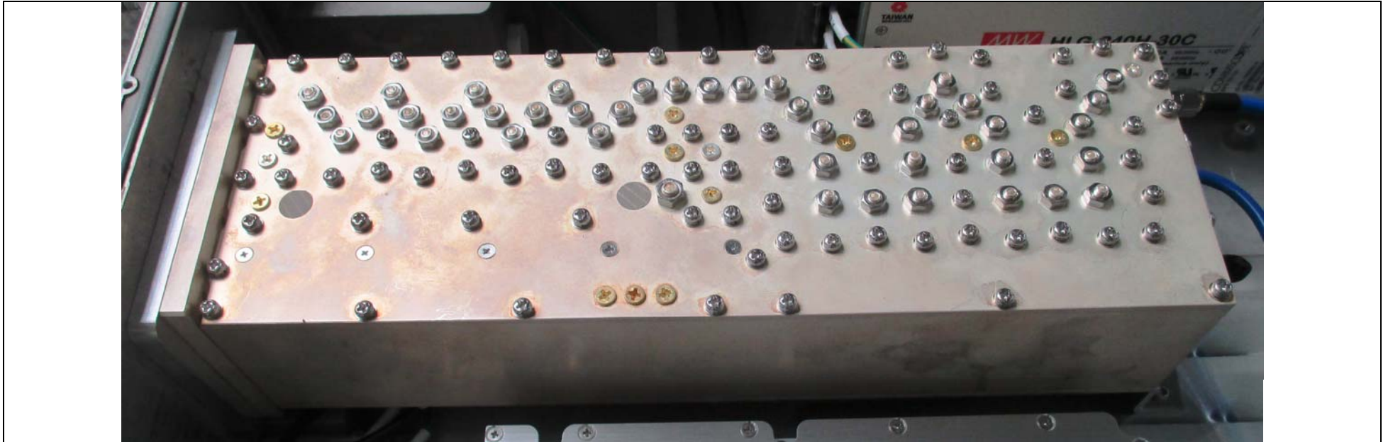
Duplexer
